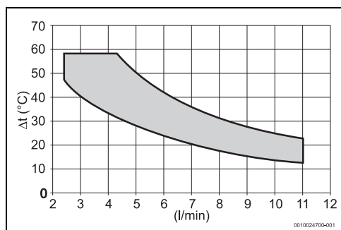
Fig. 33 Modello da 10 litri
