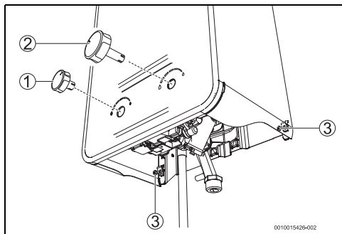
Fig. 17 Togliere il rivestimento
