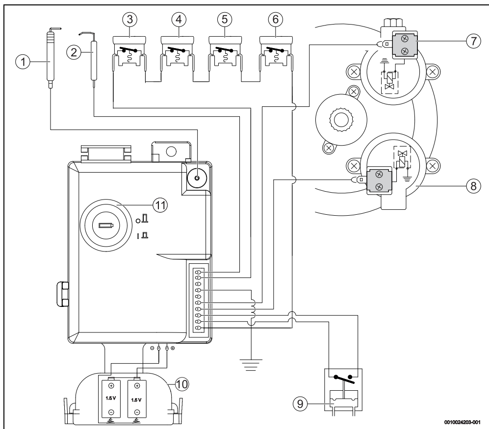
Fig. 32 Schema elettrico
