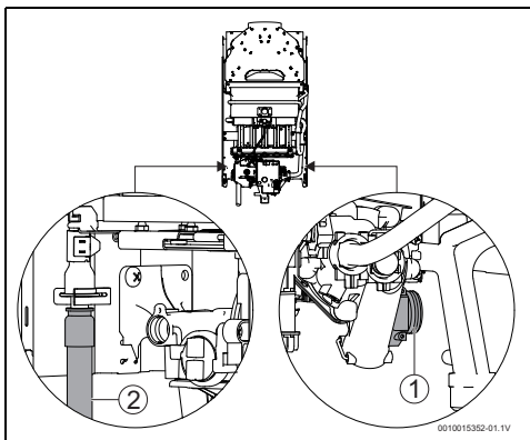
Fig. 14 Collegamento dell'acqua
