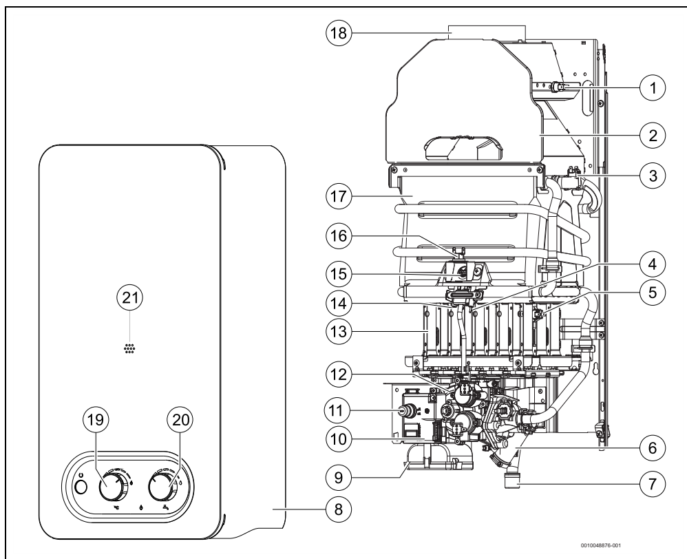
Fig. 2 Panoramica dell'apparecchio
