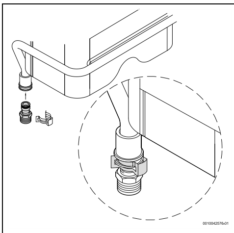
Fig. 13 Adattatore
