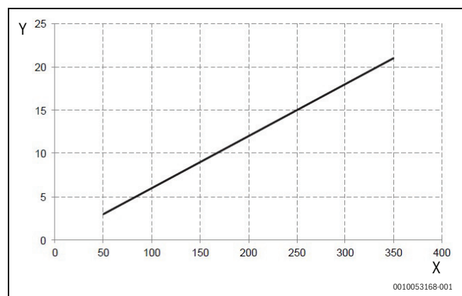
Fig. 56 Volume totale del vaso d'espansione (dimensioni da CS2000AWF 4 R-S a CS2000AWF 16 R-S/CS2000AWF 16 R-T)
