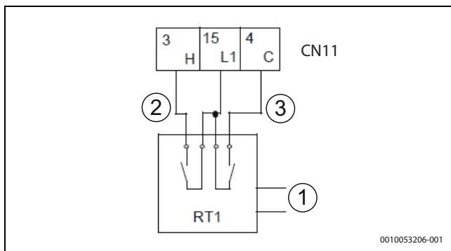
Fig. 101 Termostato di zona – metodo A
