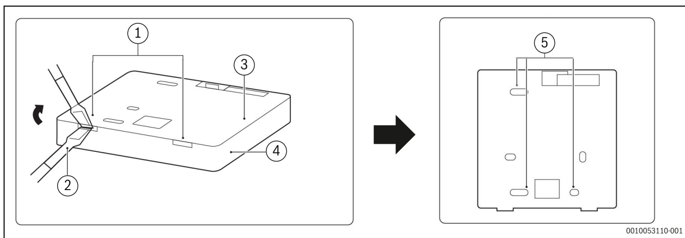
Fig. 97 Installazione a parete
