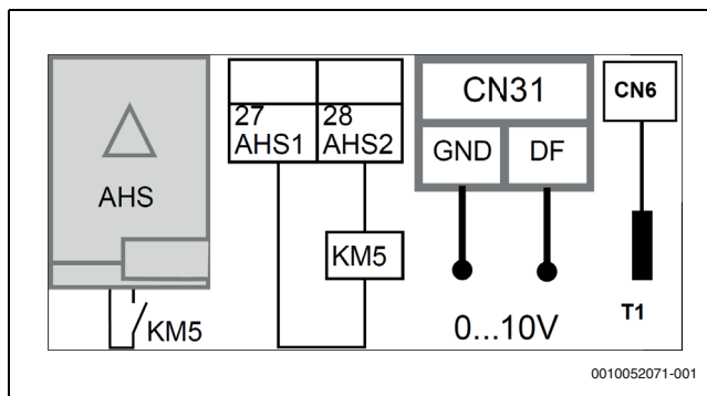
Fig. 92 Generatore di calore aggiuntivo
