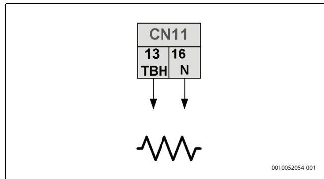
Fig. 79 Configurazione HMI cavo elettrico generatore di calore supplementare, segnale di comando tipo 2
