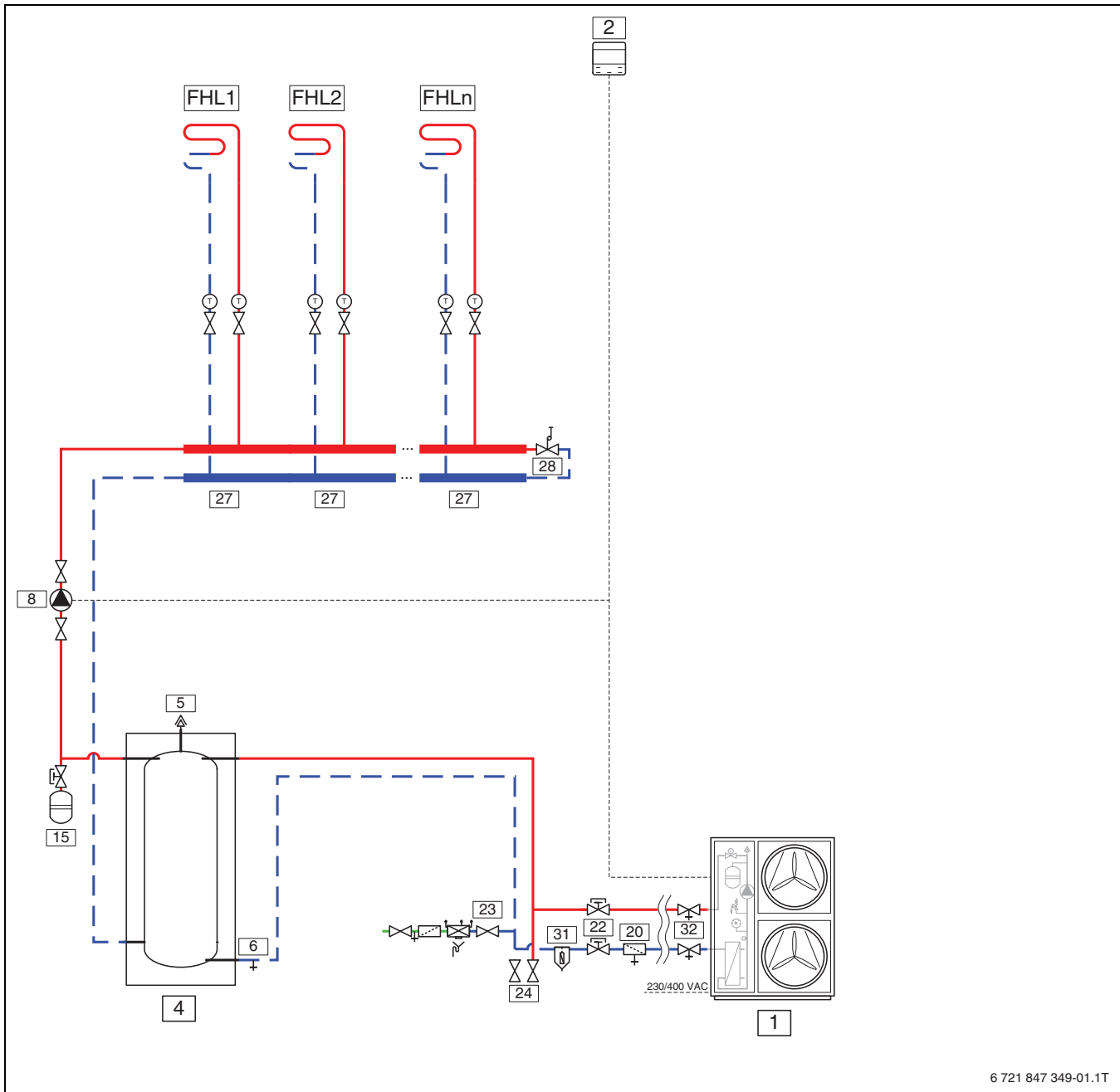
Fig. 19 Unità esterna con uno o più circuiti di riscaldamento (CS2000AWF 18-30 R-T)
