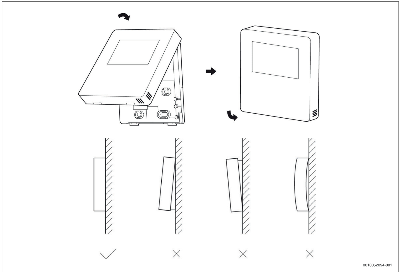
Fig. 100 Installazione del pannello anteriore
