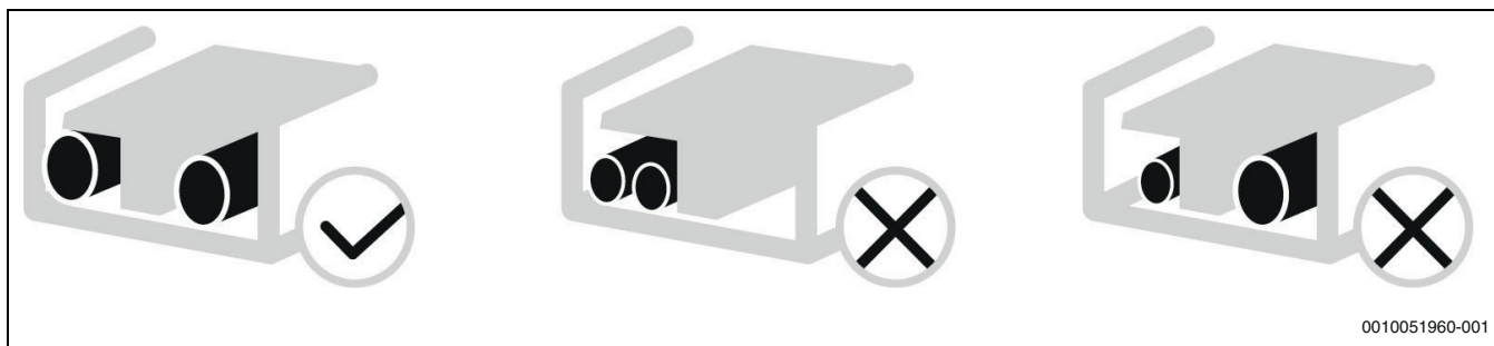
Fig. 67 Precauzioni per il collegamento dell'alimentazione elettrica
