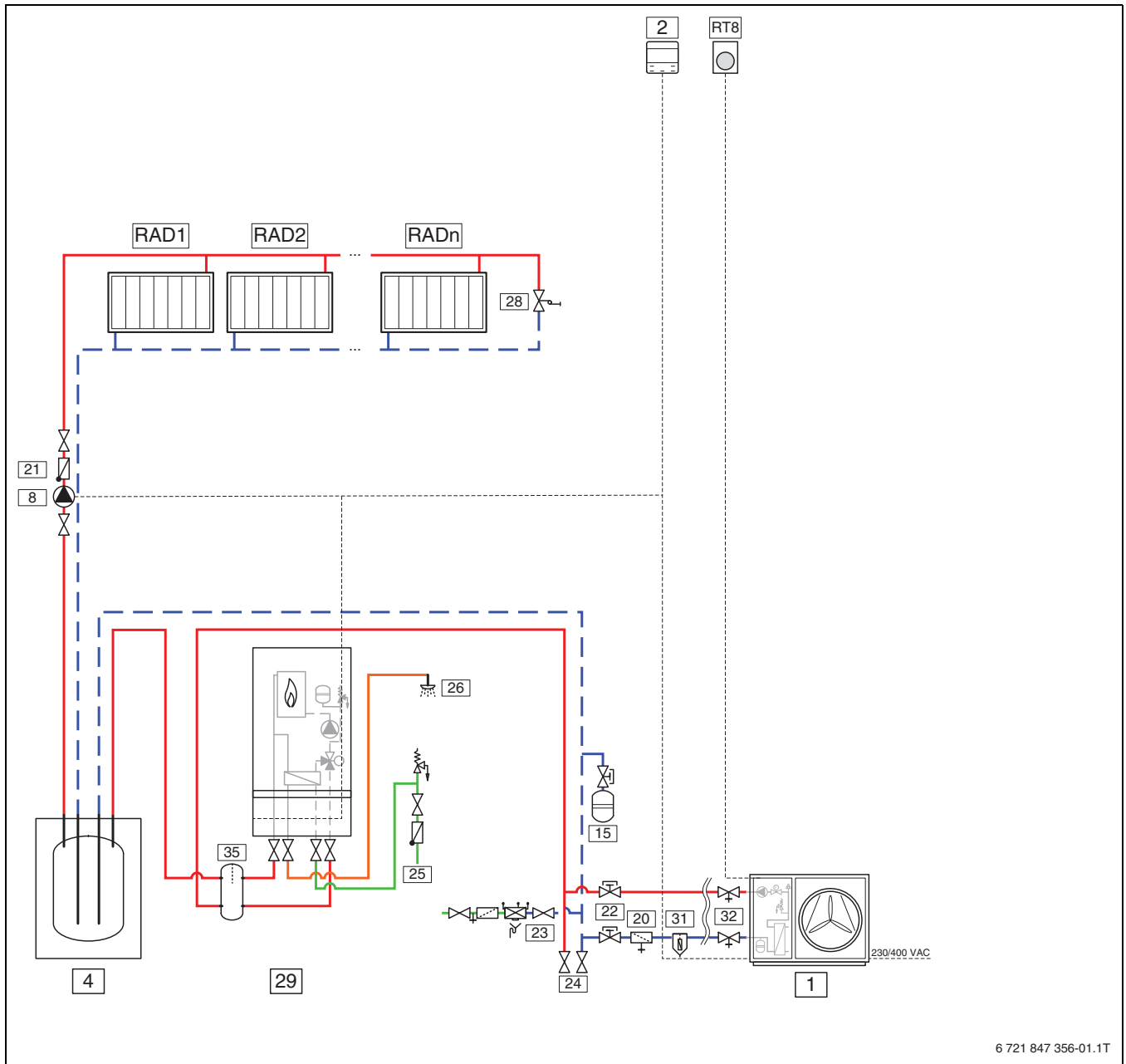
Fig. 26 Unità esterna con uno o più circuiti di riscaldamento e riscaldamento supplementare esterno (CS2000AWF 4-6 R-S, CS2000AWF 8-10 R-S, CS2000AWF 12-16 R-S/T)
