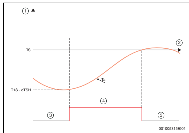
Fig. 126 Modalità riscaldamento - temperatura dell'aria ( T_a )
