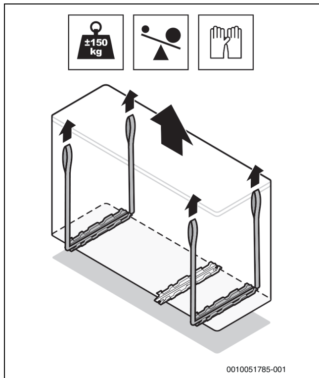
Fig. 45 Posizionamento dell'unità
