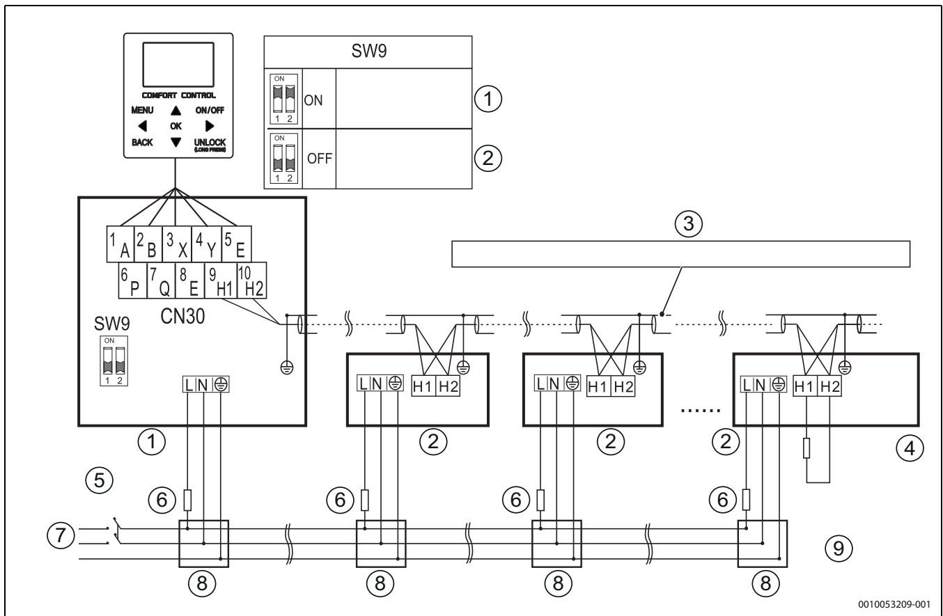
Fig. 104 Schema elettrico del sistema di regolazione elettrico per il sistema in cascata (1N~)
