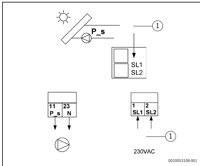
Fig. 76 Configurazione HMI sistema solare/circolatore solare
