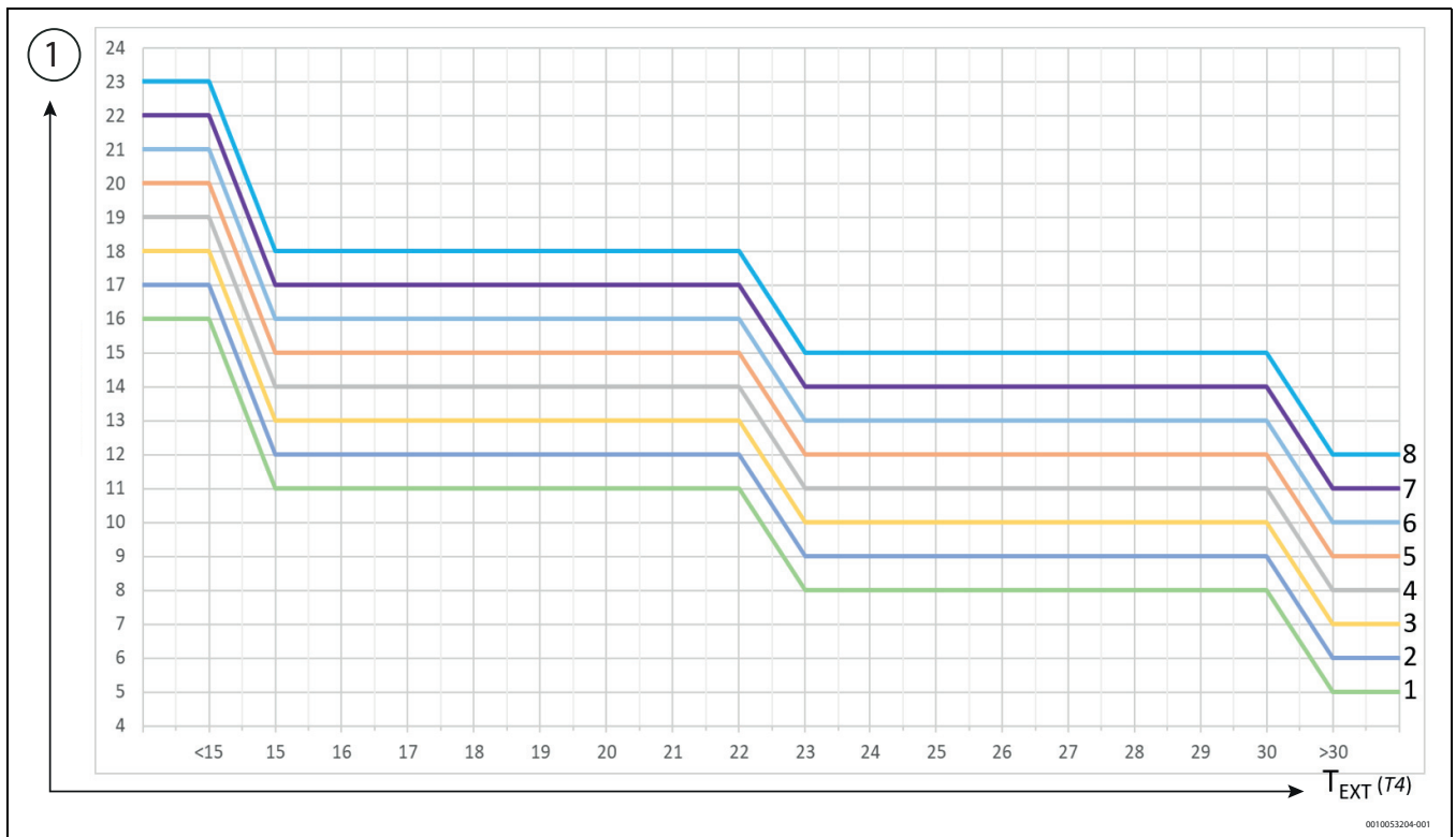
Fig. 149 Modalità raffreddamento in impianti a distribuzione terminale
