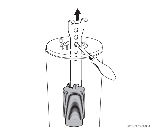
Fig. 54 Estrazione del deviatore di fiamma inferiore
