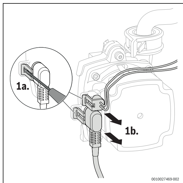
Fig. 63 Scollegamento del connettore dal circolatore riscaldamento
