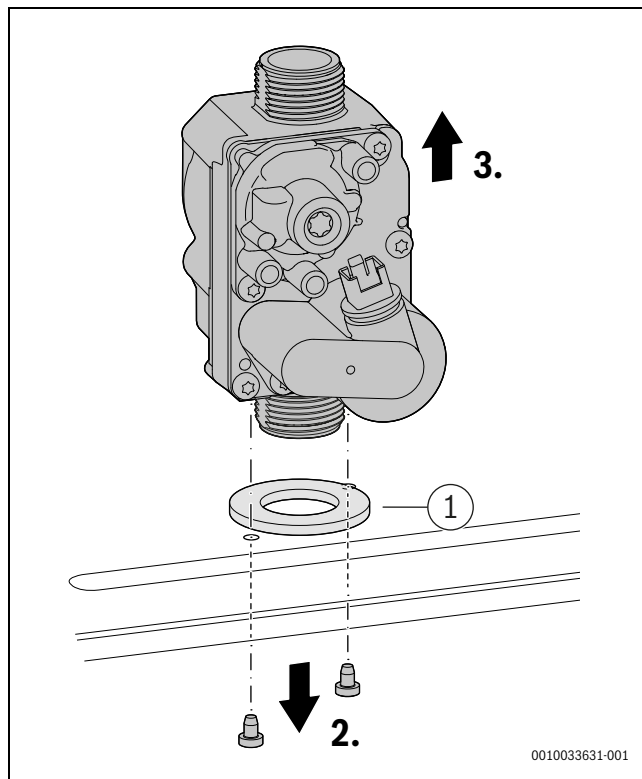
Fig. 70 Smontaggio della valvola del gas
