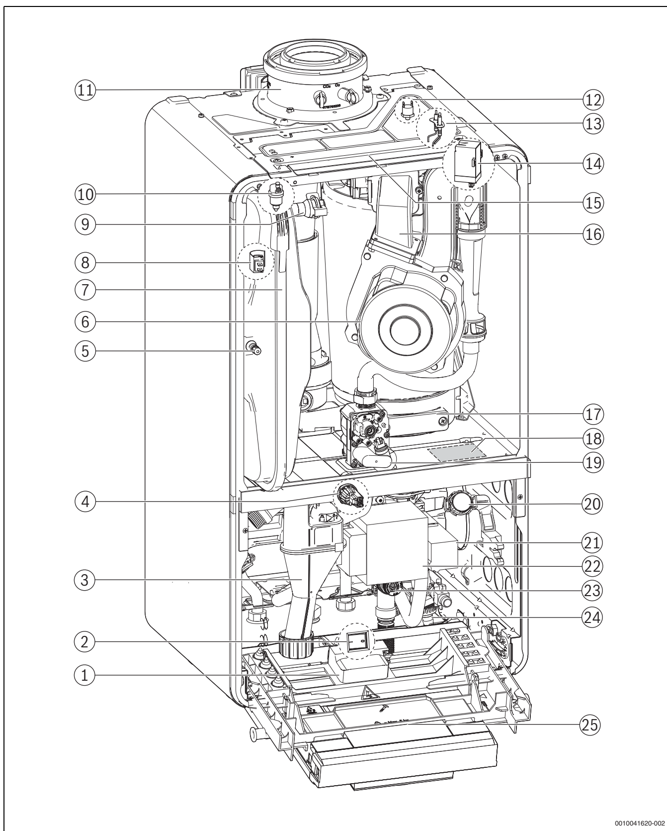
Fig. 7 Panoramica del prodotto apparecchio con bollitore
