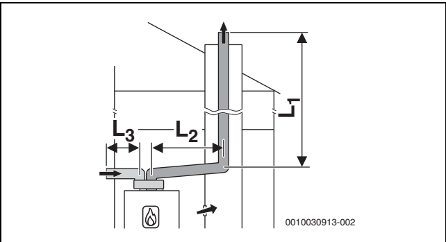
Fig. 15 Sistema di aspirazione aria/evacuazione pdc rigido secondo C 53 nel cavedio e condotto di aspirazione aria comburente/evacuazione pdc con tubi separati per adduzione aria ed evacuazione pdc nel luogo di posa
