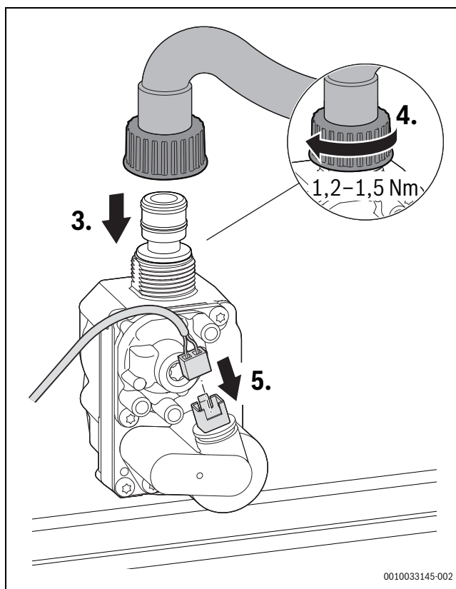
Fig. 74 Collegamento di tubo flessibile del gas e connettore – Rispettare la coppia di serraggio
