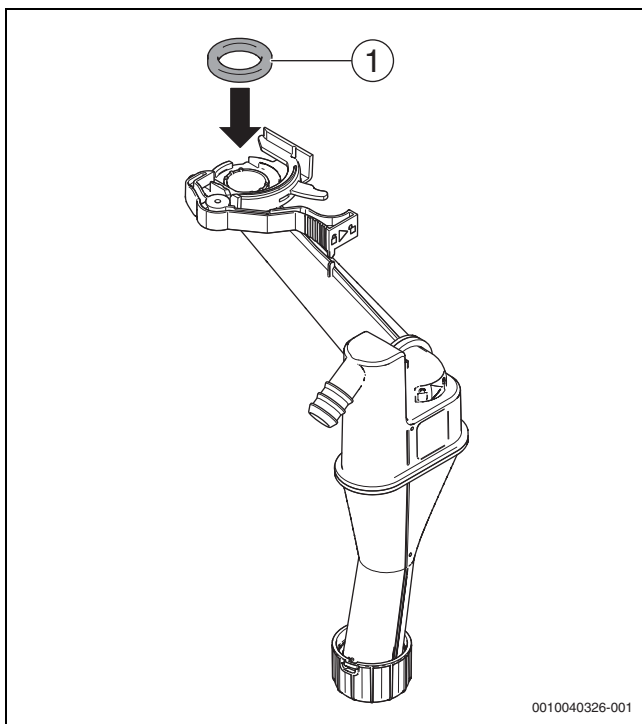
Fig. 78 Applicazione di una guarnizione nuova sul sifone per la condensa
