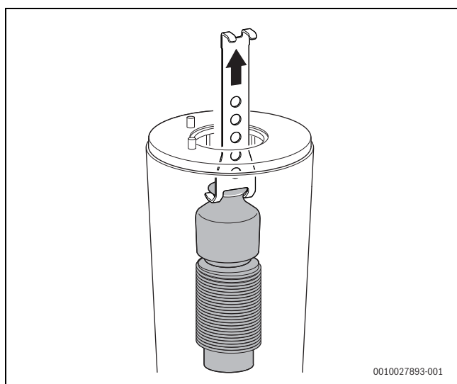
Fig. 53 Estrazione del deviatore di fiamma superiore
