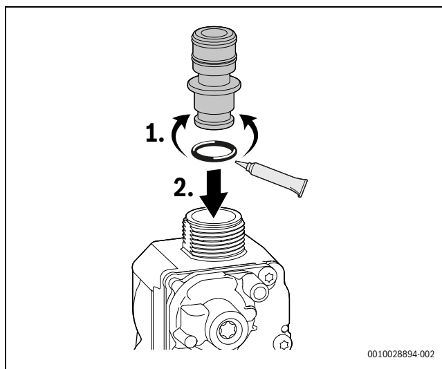
Fig. 73 Applicazione della valvola a farfalla
