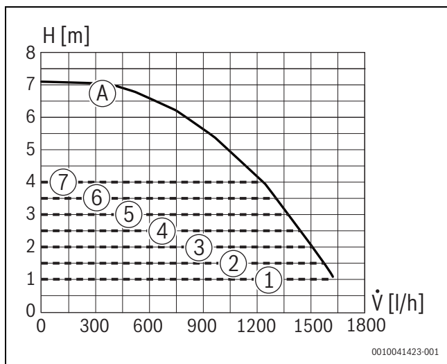
Fig. 85 Campi di lavoro del circolatore e relative curve caratteristiche
