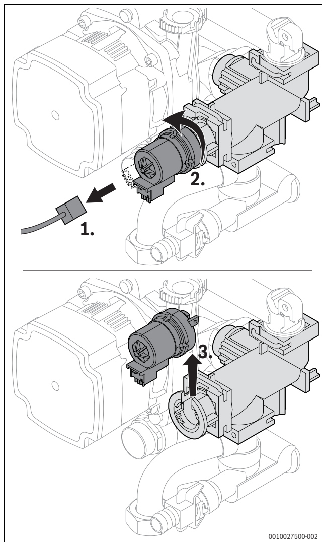
Fig. 81 Smontare il motore sulla valvola a 3 vie (variante senza viti)
