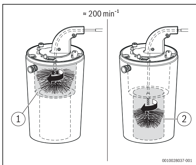
Fig. 57 Pulizia dello scambiatore primario (circa 200 min -1 , solo rotazione destrorsa)
