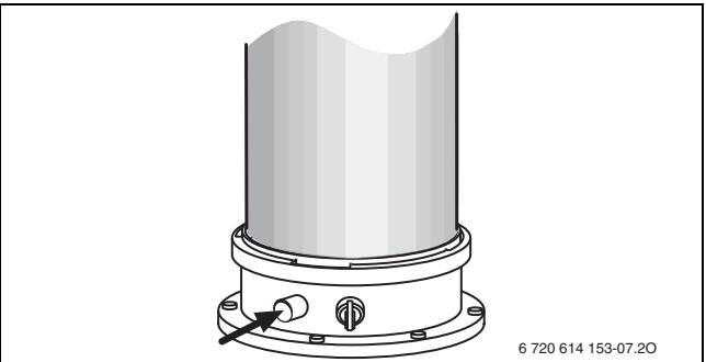
Fig. 42 Manicotto di misurazione dei gas combusti
