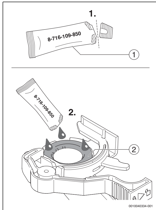
Fig. 79 Ingrassaggio della guarnizione
