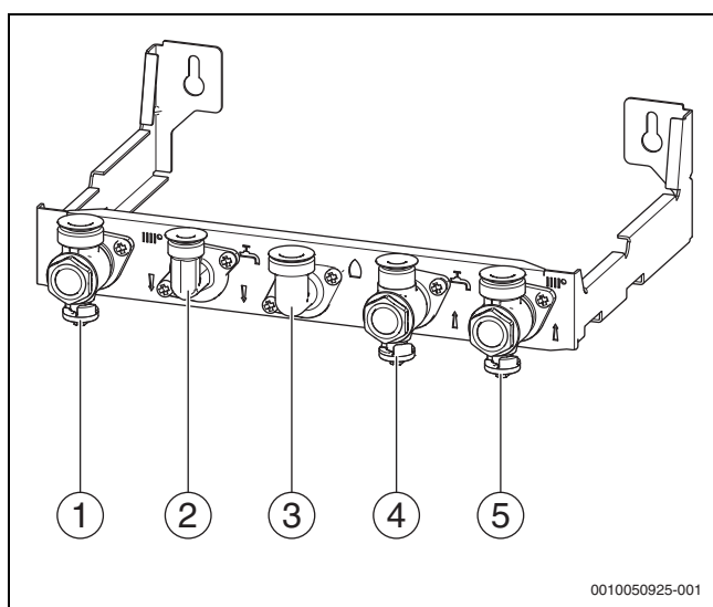
Fig. 35 Collegamenti lato gas e acqua
