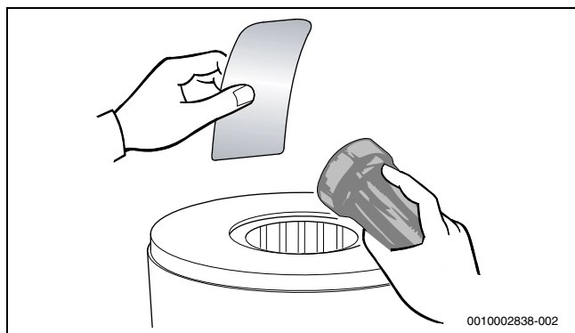
Fig. 59 Controllo della presenza di residui nello scambiatore primario
