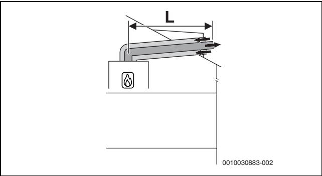
Fig. 11 Condotta di aspirazione aria comburente/evacuazione prodotti della combustione orizzontale concentrica secondo C 13x attraverso il tetto
