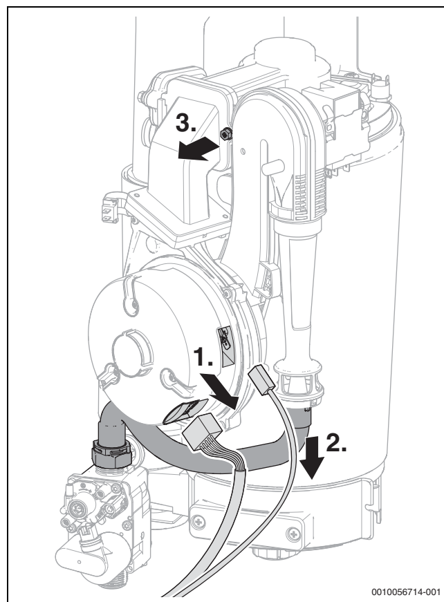
Fig. 48 Staccare il connettore e il tubo flessibile del gas, svitare la vite
