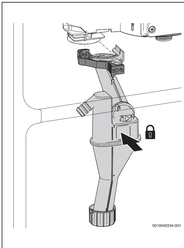
Fig. 80 Applicazione del sifone per la condensa
