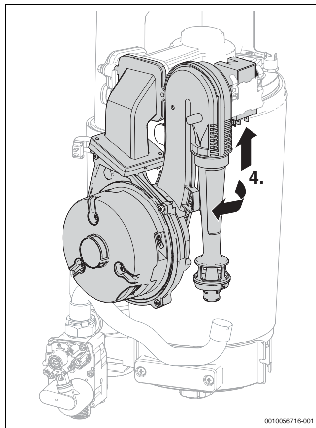
Fig. 49 Rimuovere il tubo di venturi con il miscelatore e il ventilatore
