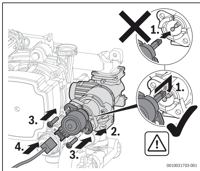
Fig. 84 Montare il motore sulla valvola a 3 vie (variante con viti)
