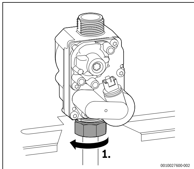
Fig. 69 Svitamento del dado a risvolto
