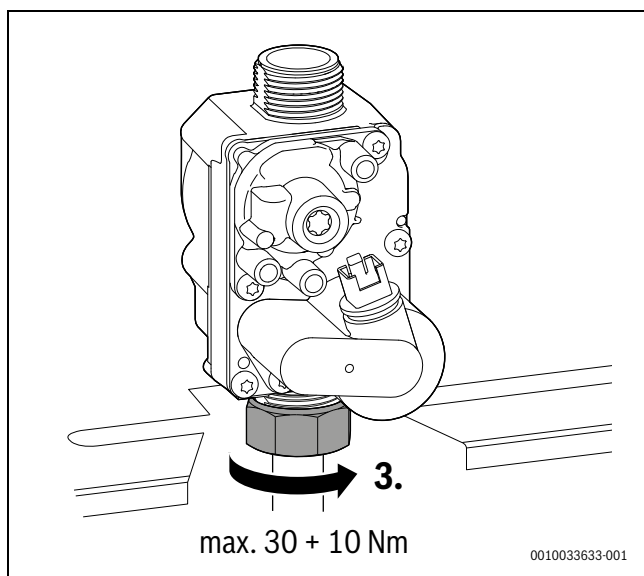
Fig. 72 Rispettare la coppia di serraggio
