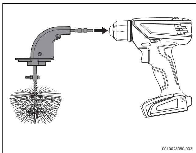
Fig. 56 Montaggio della spazzola sull'avvitatore a batteria
