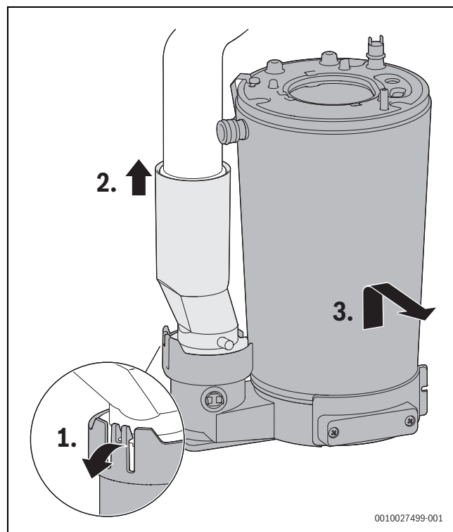
Fig. 62 Smontaggio dello scambiatore primario
