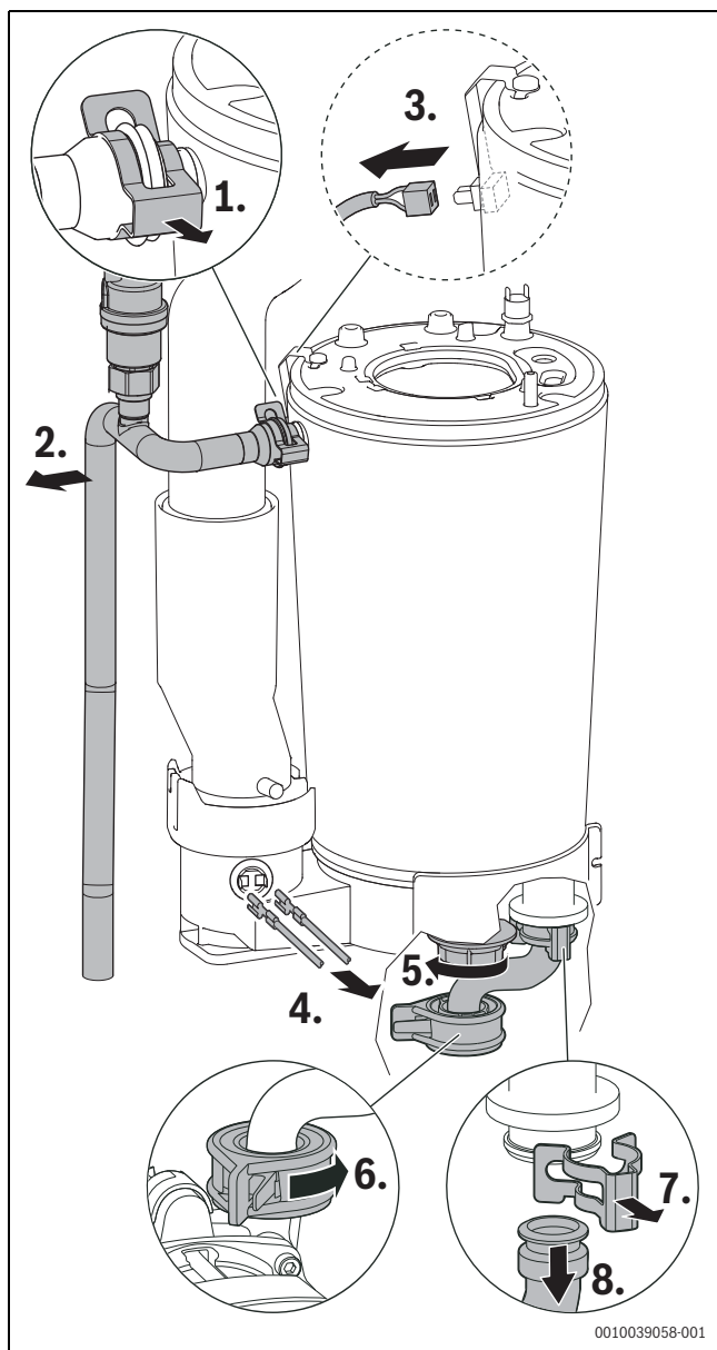
Fig. 61 Scollegamento di tubo di mandata, cavo conduttore e tubo di ritorno
