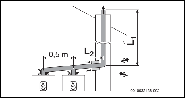
Fig. 26 Impianto a cascata con 2 apparecchi: sistema di aspirazione aria comburente/evacuazione dei prodotti della combustione rigido nel cavedio secondo B 53p con adduzione aria comburente sull'apparecchio dipendente dall'aria del locale
