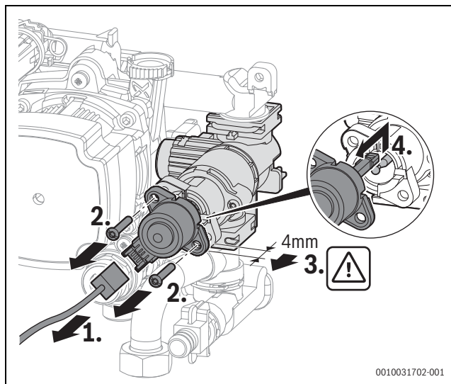
Fig. 83 Smontare il motore sulla valvola a 3 vie (variante con viti)
