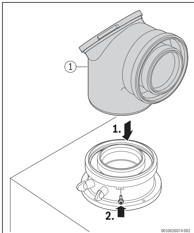
Fig. 34 Applicare l'accessorio del sistema aspirazione aria / evacuazione prodotti della combustione e fissarlo con la vite
