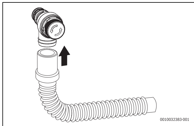
Fig. 31 Montare il tubo flessibile alla valvola di sicurezza del riscaldamento
