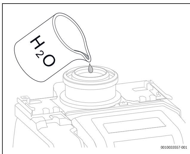
Fig. 33 Riempimento del sifone per la condensa con acqua
