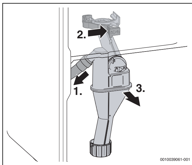
Fig. 76 Smontaggio del sifone per la condensa
