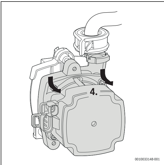
Fig. 65 Rimozione del circolatore riscaldamento
