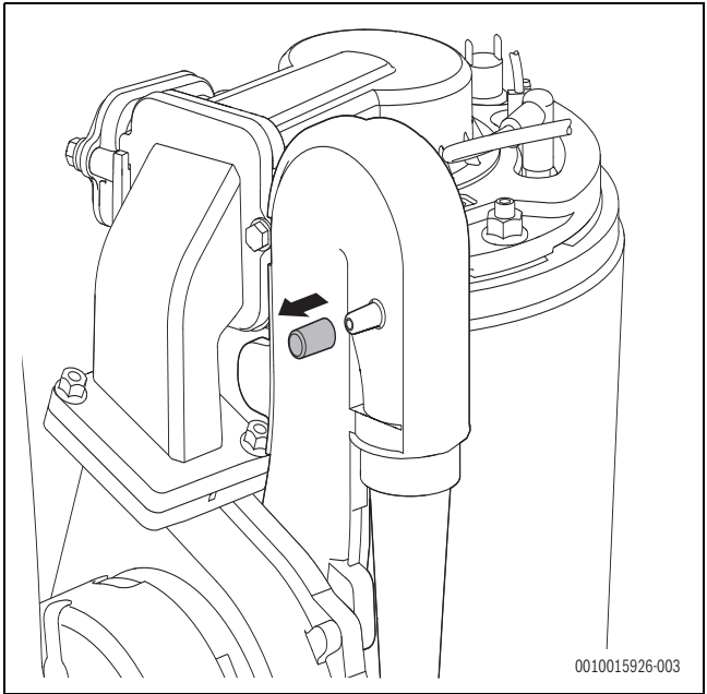
Fig. 46 Manicotto di misurazione sul miscelatore
