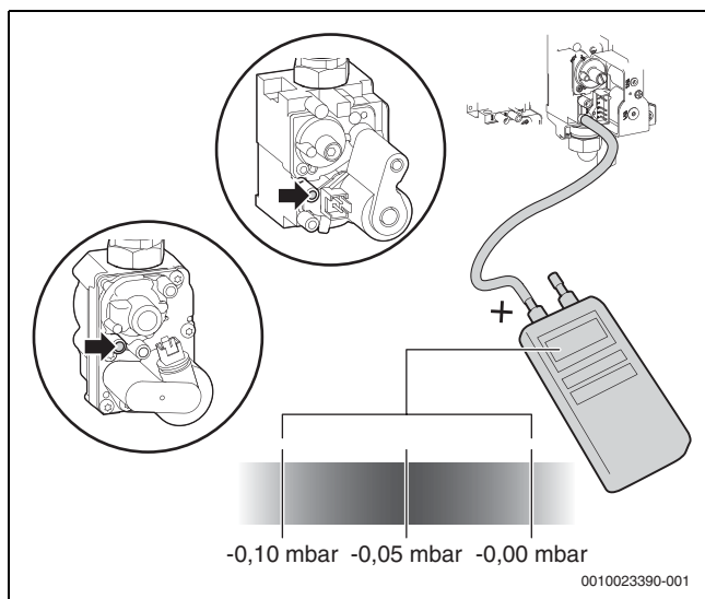
Fig. 43 Misurare la pressione differenziale
