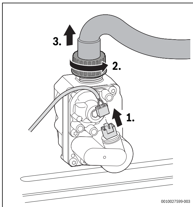
Fig. 67 Scollegamento del connettore dalla valvola del gas e rimozione del dado a risvolto con il tubo flessibile del gas
