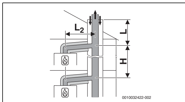
Fig. 24 Collettore scarico gas combusto secondo C_{(14)3x} con sistema di aspirazione aria comburente/evacuazione prodotti della combustione collettivo concentrico e condotto di aspirazione aria comburente/evacuazione prodotti della combustione concentrico nel luogo di posa
