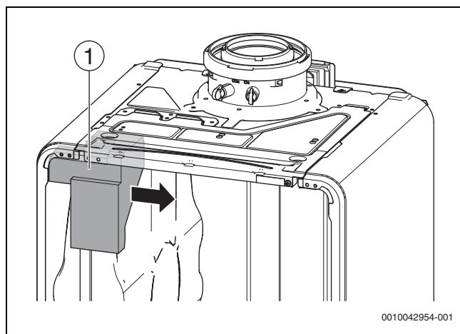
Fig. 30 Rimozione della resina espansa
