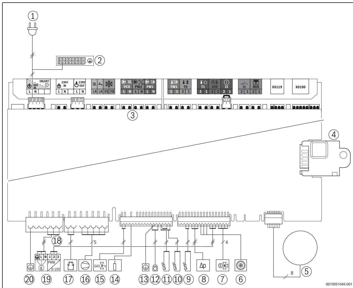
Fig. 86 Cablaggio elettrico
