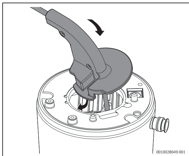
Fig. 55 Introduzione della spazzola nello scambiatore primario
