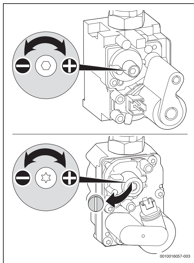
Fig. 44 Taratura della valvola del gas
