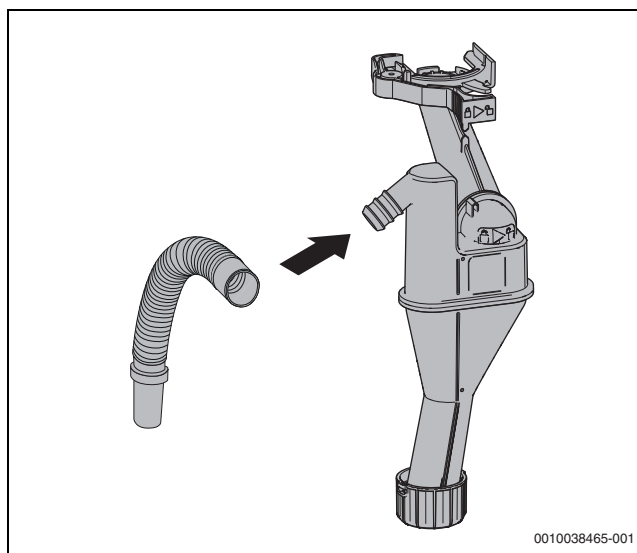
Fig. 32 Innesto del tubo flessibile per scarico condensa sul raccordo
