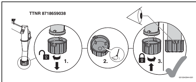
Fig. 77 Pulizia del dispositivo di ritenzione impurità
