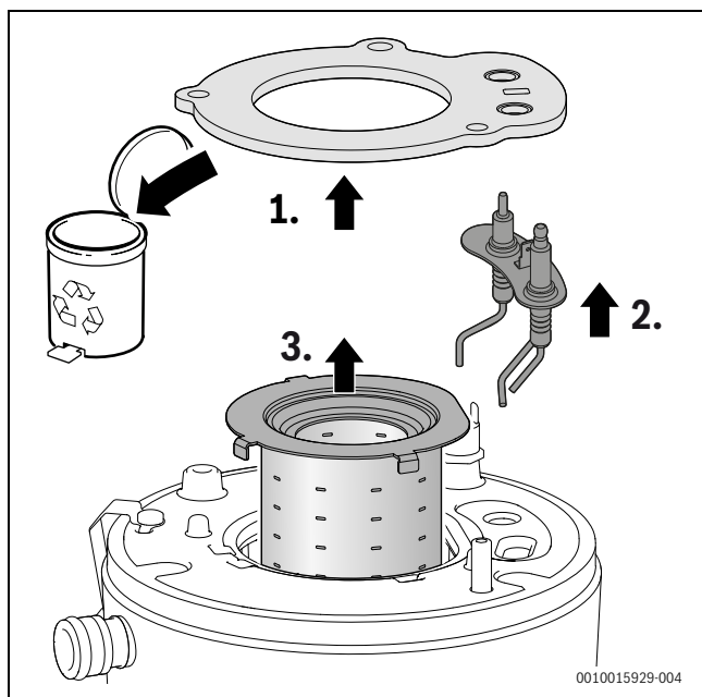
Fig. 52 Estrazione del bruciatore
