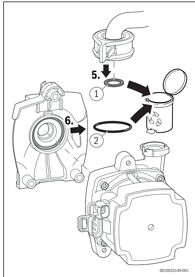
Fig. 66 Smaltimento delle guarnizioni
