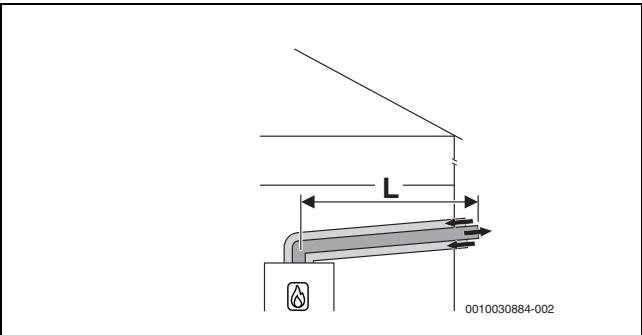
Fig. 10 Condotta di aspirazione aria comburente/evacuazione pdc orizzontale concentrica secondo C 13x attraverso la parete esterna
