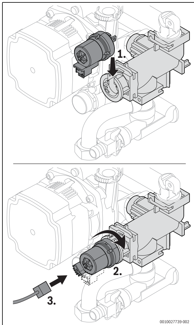
Fig. 82 Montare il motore sulla valvola a 3 vie (variante senza viti)
