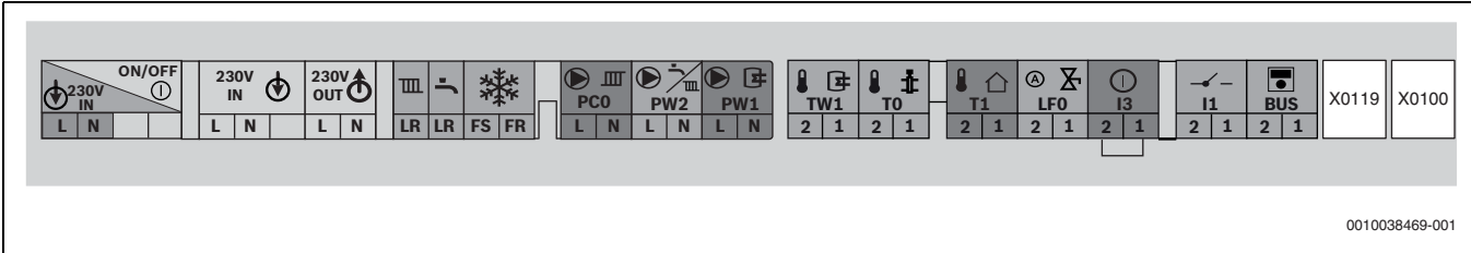
Fig. 38 Morsettiera per accessorio esterno
