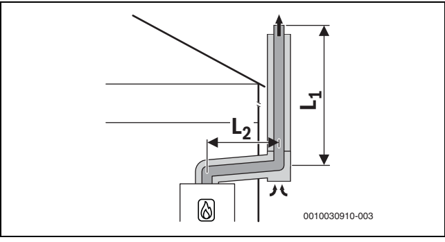
Fig. 17 Condotto di aspirazione aria comburente/evacuazione prodotti della combustione concentrico secondo C 53x sulla parete esterna
