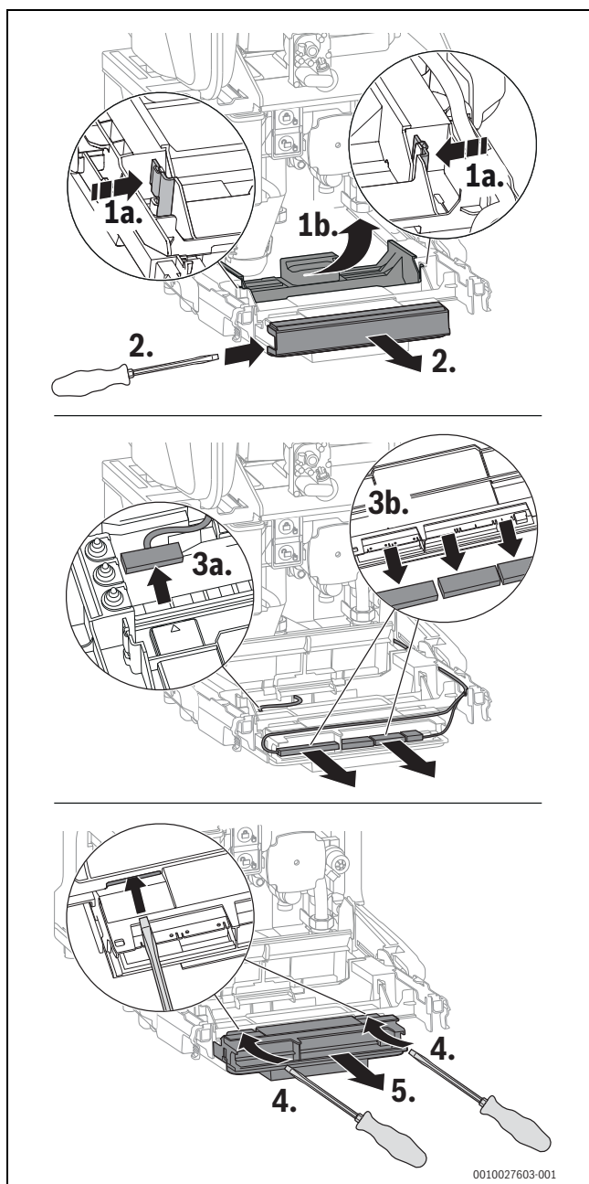
Fig. 75 Rimozione del dispositivo di controllo
