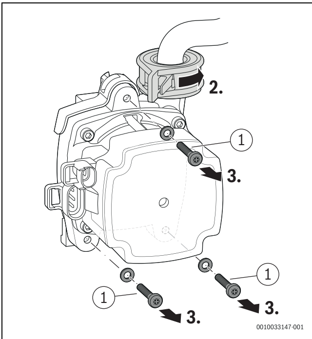
Fig. 64 Sbloccaggio del circolatore riscaldamento e rimozione delle viti
