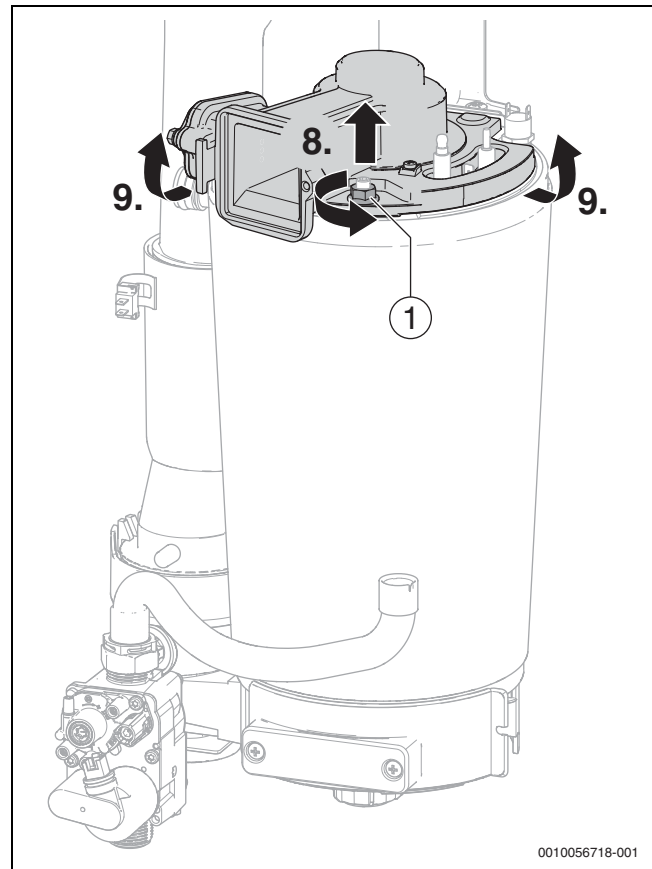
Fig. 51 Rimozione del coperchio del bruciatore con ventilatore e miscelatore
