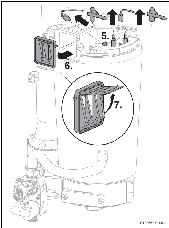
Fig. 50 Scollegamento dei cavi
