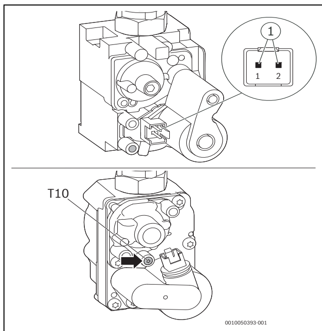
Fig. 47 Punti di misurazione sulla valvola del gas
