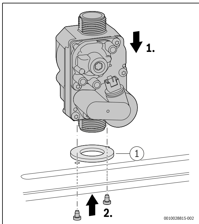
Fig. 71 Montaggio della valvola del gas
