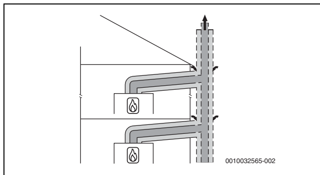
Fig. 23 Collettore scarico gas combusto secondo C_{(12)3x} con condotto di aspirazione aria comburente/evacuazione prodotti della combustione concentrico nel luogo di posa
