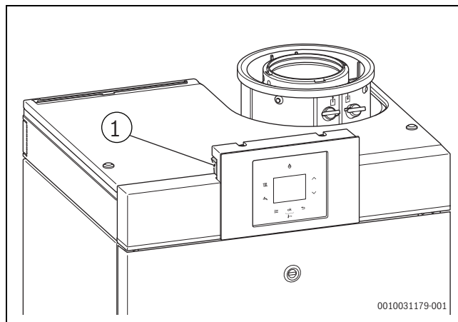
Fig. 5 Interruttore on/off
