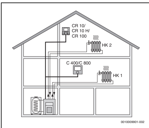
Fig. 2 CR 10/CR 10 H/CR 100 come termoregolatore ambiente per il secondo circuito di riscaldamento (HK 2) e C 400/C 800 come termoregolatori e per il primo circuito di riscaldamento (HK 1)
