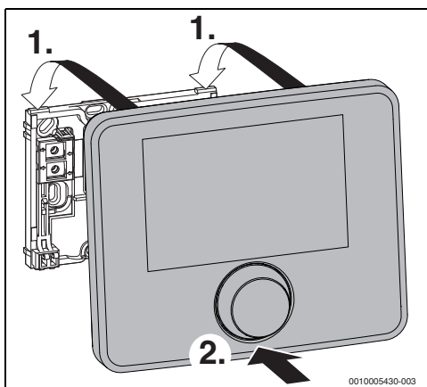
Fig. 8 Agganciare il termoregolatore
