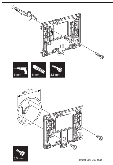
Fig. 6 Montaggio della basetta di supporto per installazione a parete
