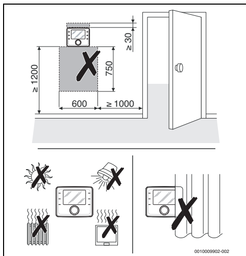
Fig. 5 Luogo di installazione nel locale di riferimento
