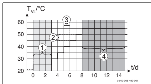
Fig. 20 Esecuzione dell'asciugatura massetto con le impostazioni di fabbrica nella fase di riscaldamento
