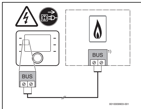
Fig. 7 Collegamento del termoregolatore al generatore di calore
