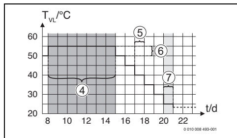
Fig. 21 Esecuzione dell'asciugatura massetto con le impostazioni di fabbrica nella fase di raffreddamento
