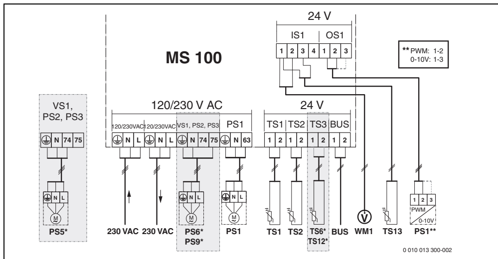
Afb. 1 Bezetting aansluitklemmen voor zonnesysteem
