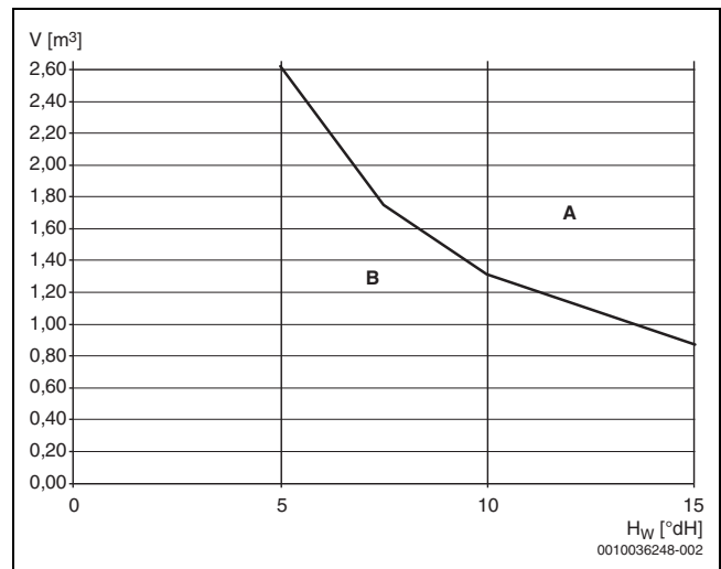
Fig. 1 Valori limite per il trattamento dell'acqua degli impianti a pompa di calore
