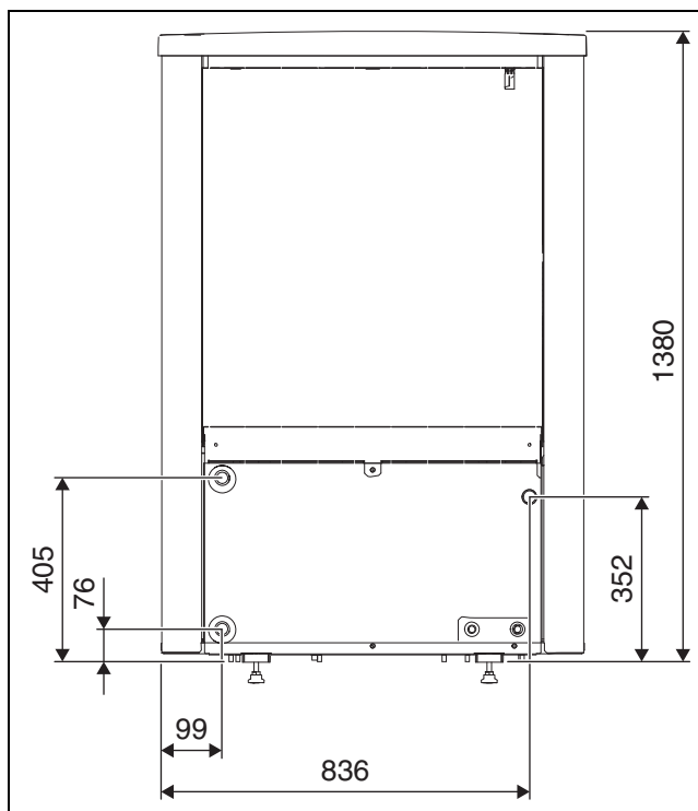
Fig. 4 Dimensioni e attacchi del modello di pompa di calore 5-9, lato posteriore
