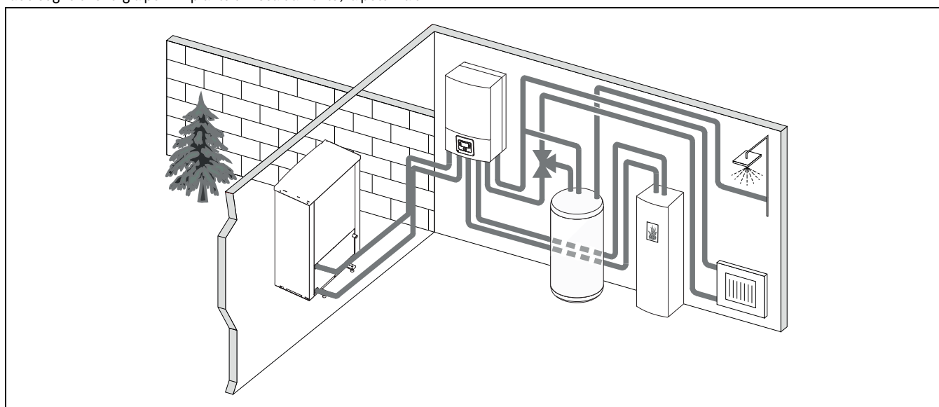
Fig. 3 Pompa di calore Compress 6000 AW, unità interna AWB senza resistenza elettrica supplementare, bollitore ACS esterno e generatore di calore supplementare esterno
