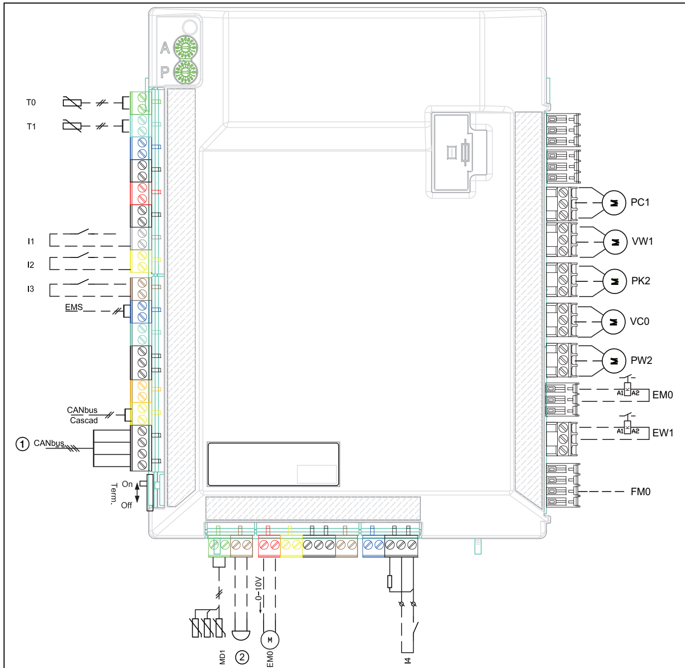
Fig. 12 Collegamenti modulo di installazione
