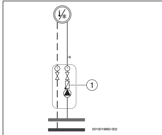
Fig. 30 Circuito di riscaldamento
