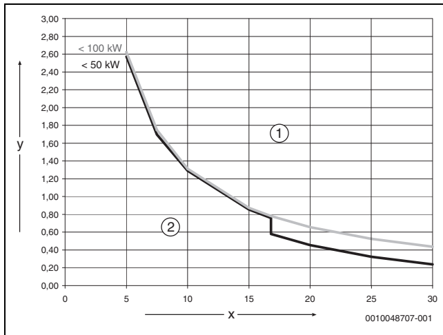
Fig. 1 Generatore di calore < 50 kW < 100 kW
