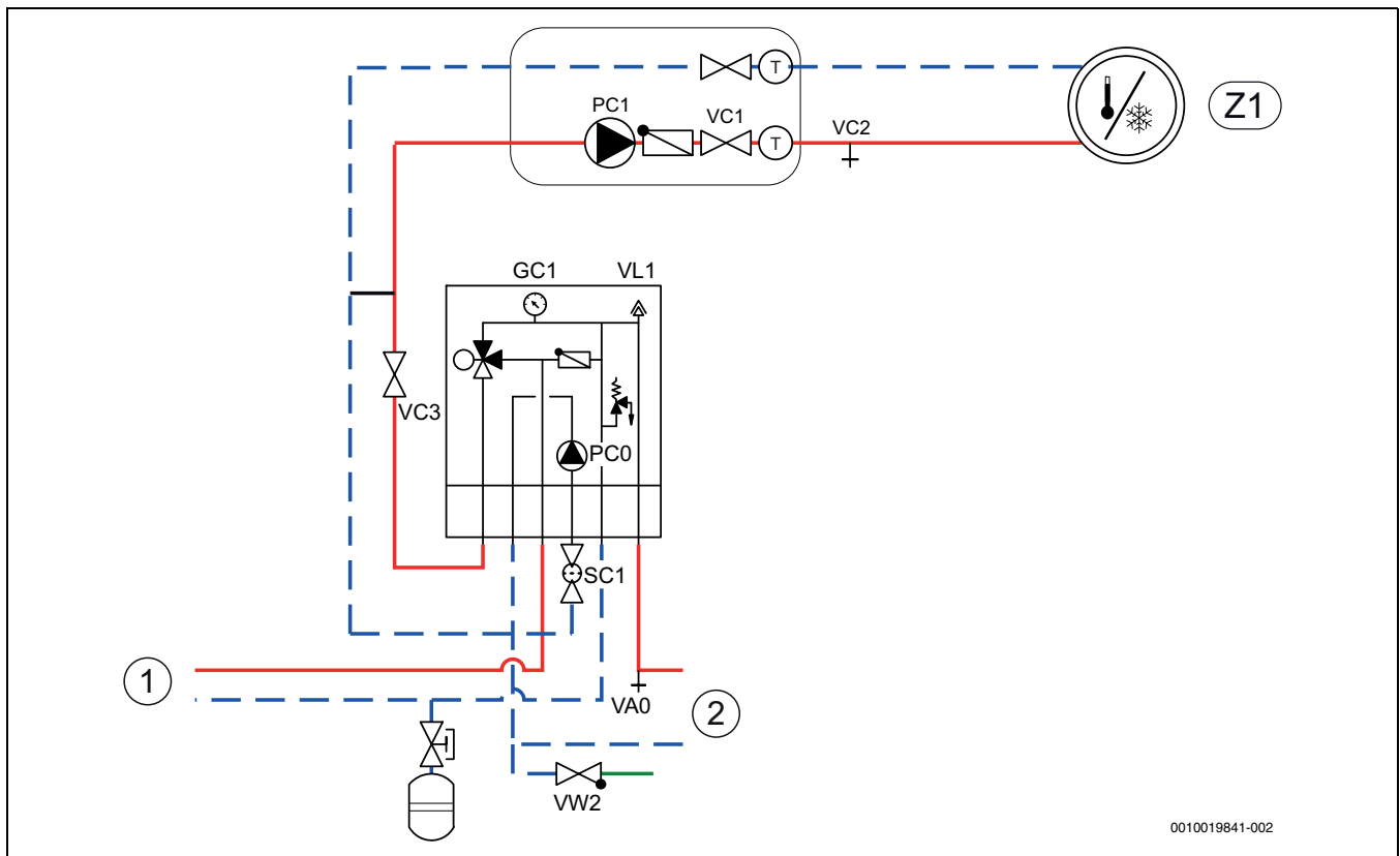
Fig. 19 Unità interna con generatore di calore esterno supplementare e sistema di riscaldamento
