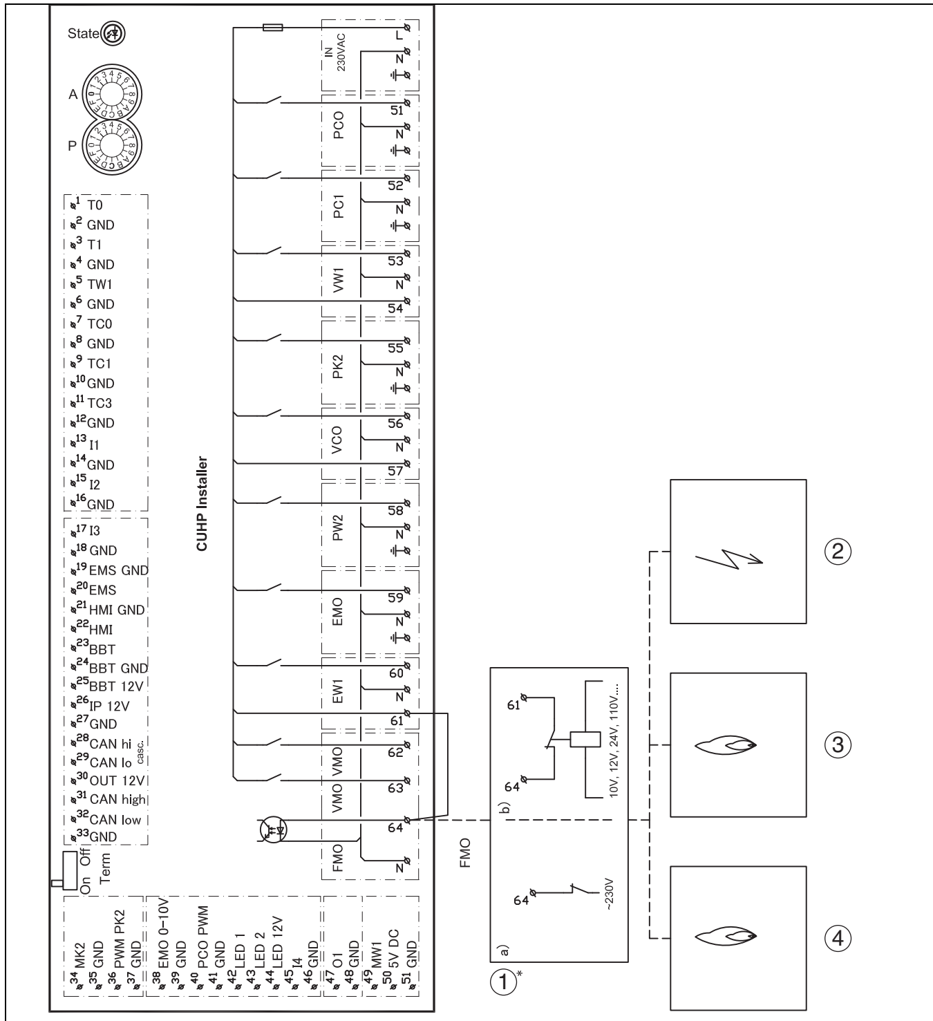
Fig. 37 Schema elettrico per il modulo di installazione, allarme del generatore di calore esterno supplementare
