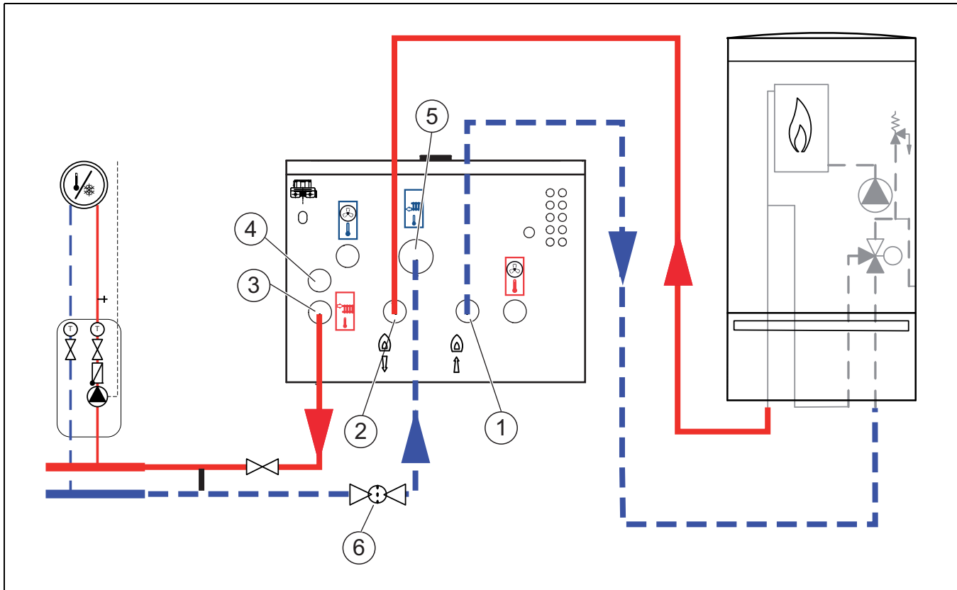
Fig. 7 Collegamento dell'unità interna con valvola miscelatrice per generatore di calore esterno supplementare all'impianto di riscaldamento e al generatore di calore esterno supplementare
