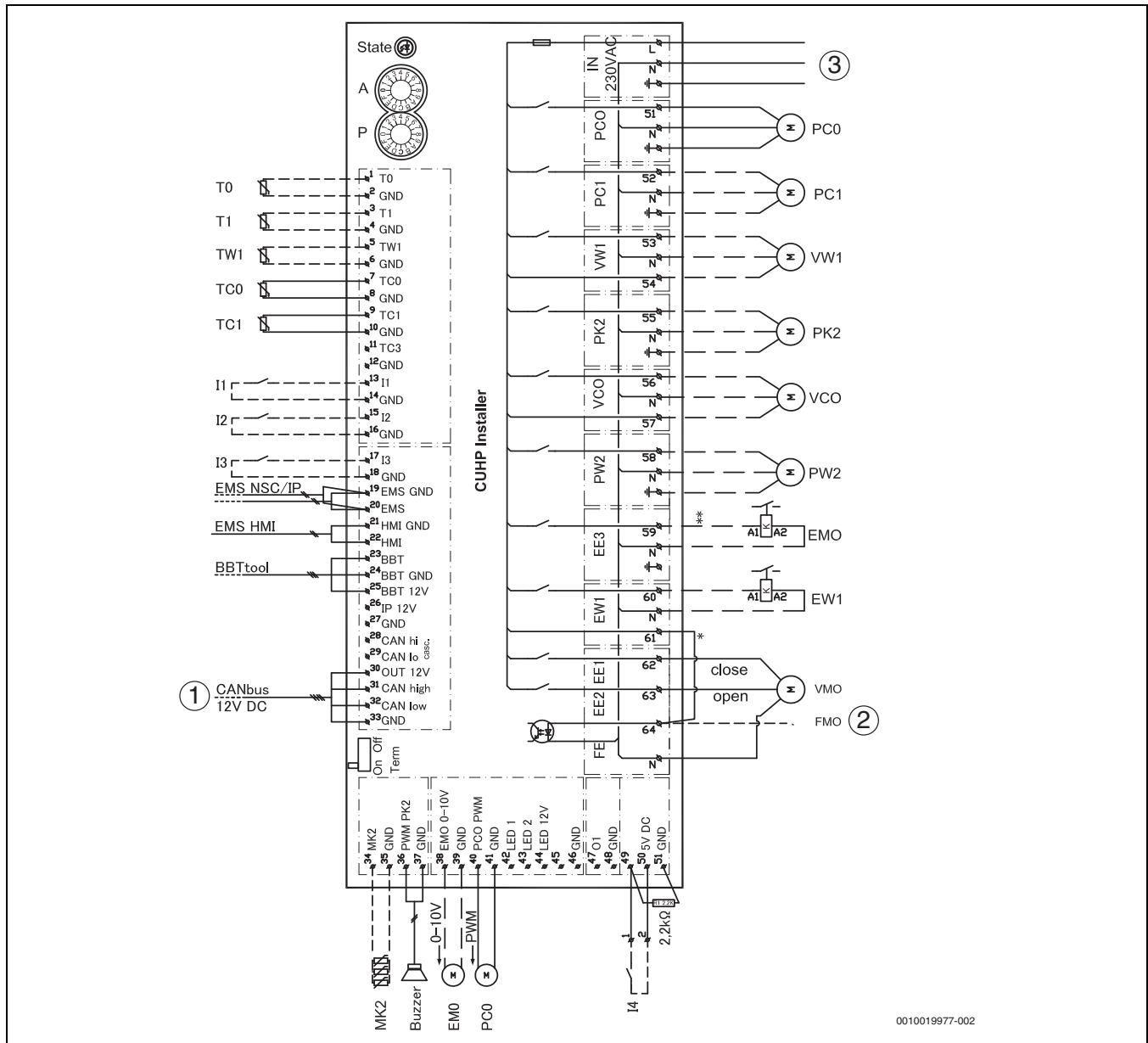
Fig. 35 Schema elettrico modulo di installazione per unità interna con valvola miscelatrice per generatore di calore esterno supplementare
