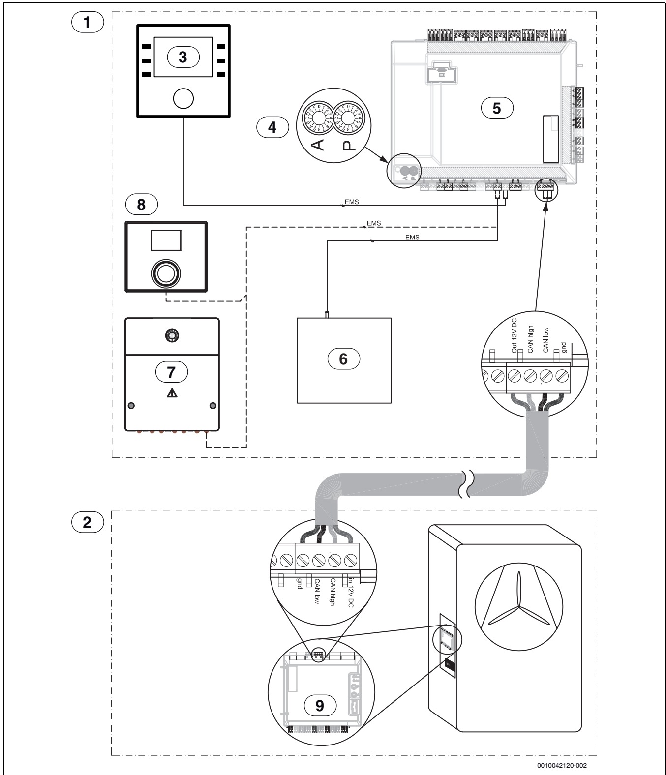
Fig. 32 Unità interna con valvola miscelatrice per riscaldatore esterno supplementare – panoramica CAN-/EMS-BUS
