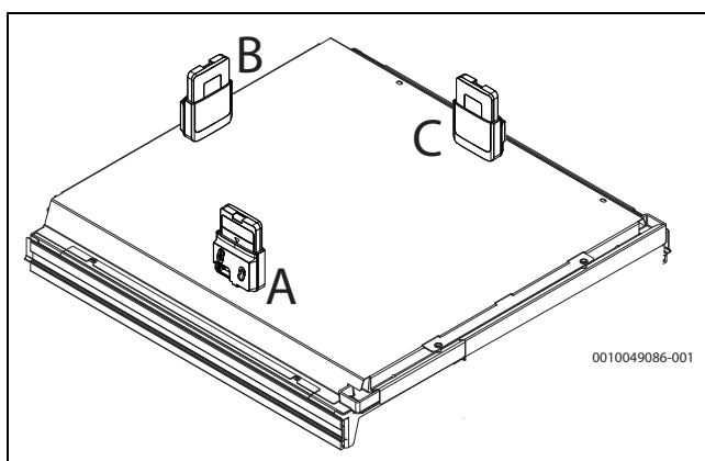
Fig. 16 Applicare il supporto sul pannello di copertura superiore dell'unità interna. In aggiunta al supporto, la figura mostra anche il Modulo wireless all'interno del supporto
