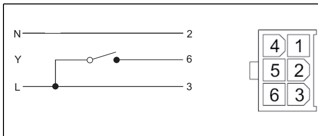
Fig. 26 Connettore Molex
