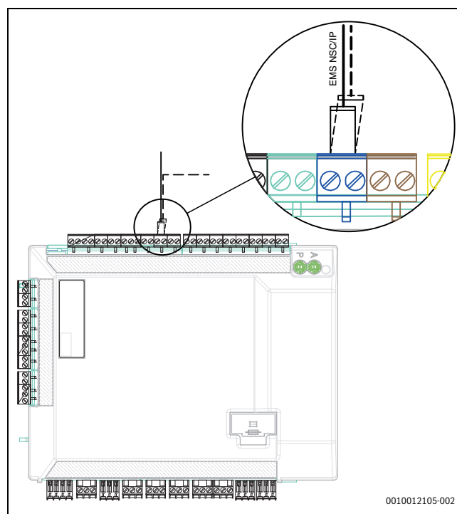
Fig. 21 Collegamento EMS nel modulo di installazione
