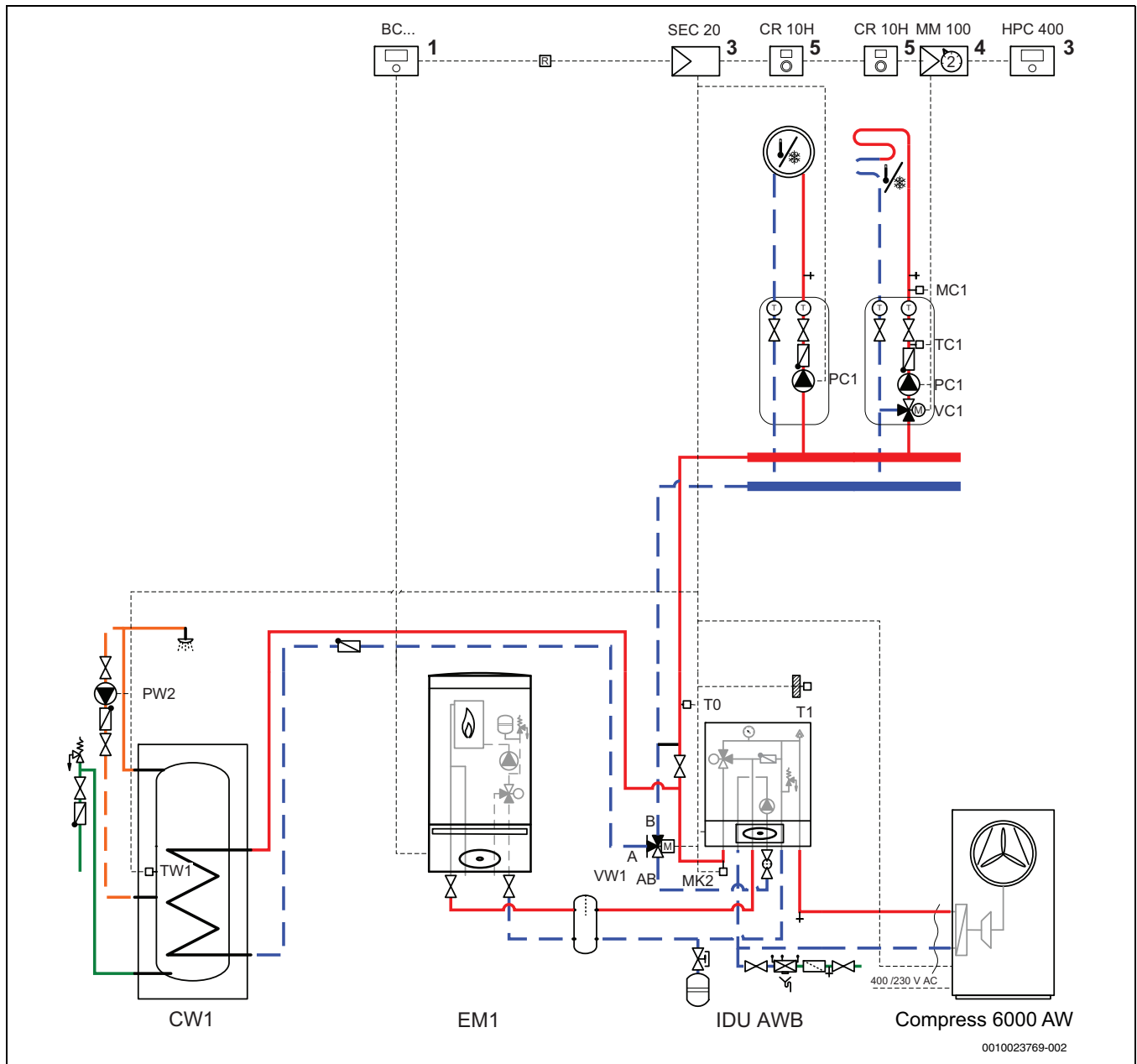
Fig. 31 Generatore di calore supplementare con valvola miscelatrice e bollitore d'acqua calda sanitaria
