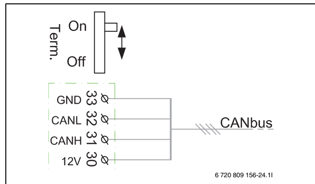
Fig. 9 Terminazione CAN-BUS
