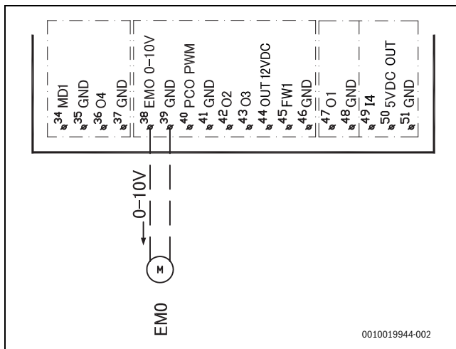
Fig. 13 Comando da 0 a 10 V per generatori di calore esterni supplementari
