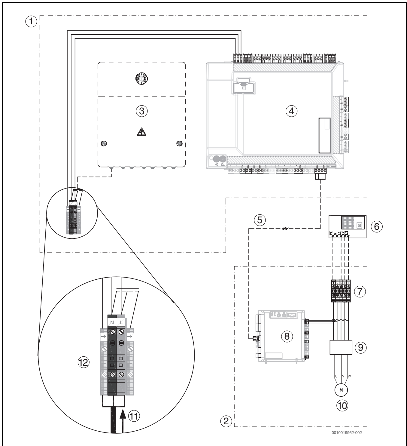
Fig. 34 Pompa di calore trifase e unità interna con generatore di calore esterno supplementare
