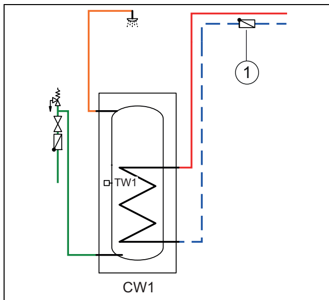
Fig. 22 Bollitore d'acqua calda sanitaria
