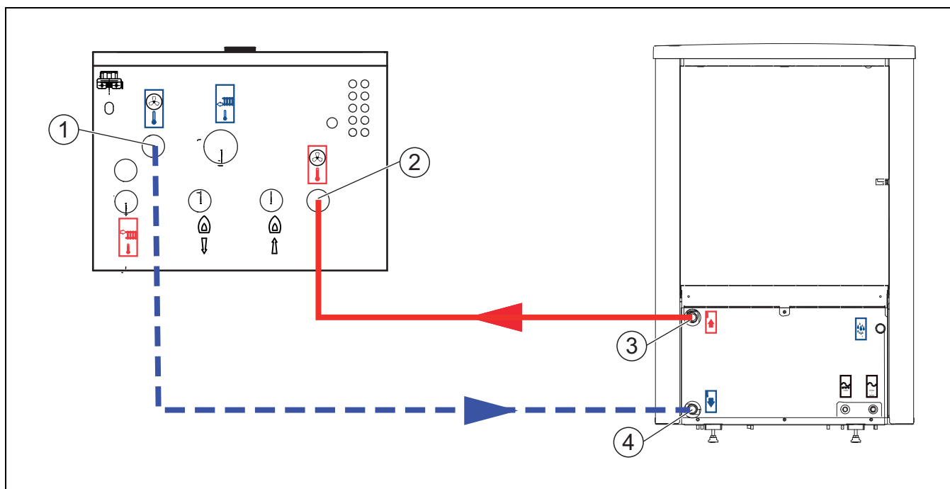
Fig. 6 Collegamento dell'unità interna alla pompa di calore
