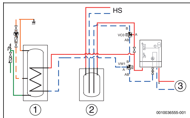
Fig. 28 Accumulatore inerziale, valvola bypass VCO
