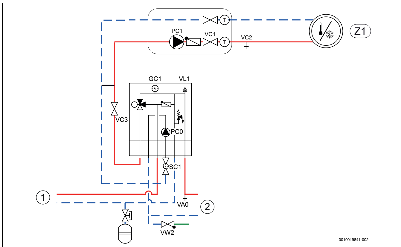
Fig. 8 Unità interna con generatore di calore esterno supplementare e sistema di riscaldamento
