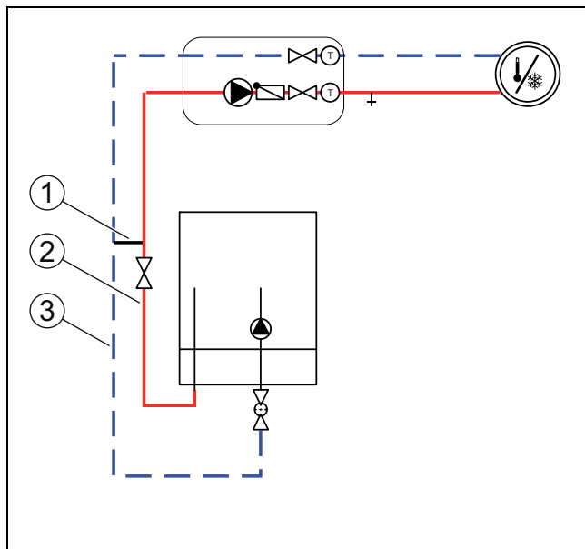
Fig. 29 Unità interna con circuito di riscaldamento e bypass
