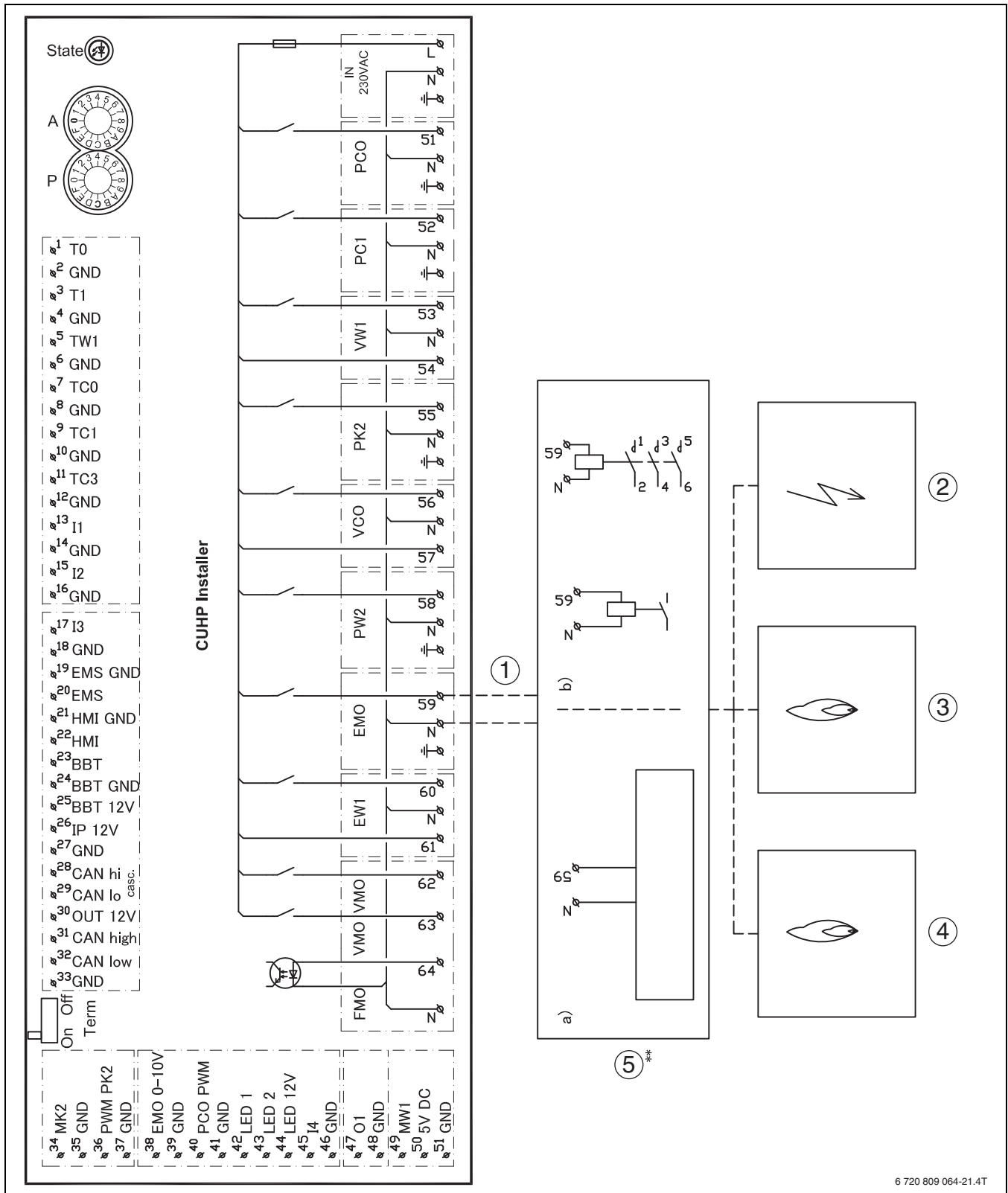
Fig. 36 Schema elettrico per modulo di installazione, accensione/spengimento con generatore di calore esterno supplementare
