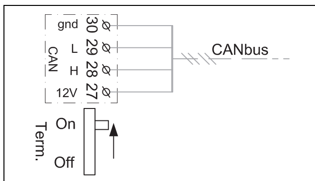
Fig. 16 Terminazione CAN-BUS
