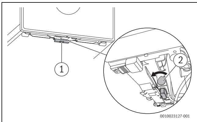
Fig. 5 Messa in sicurezza della Key
