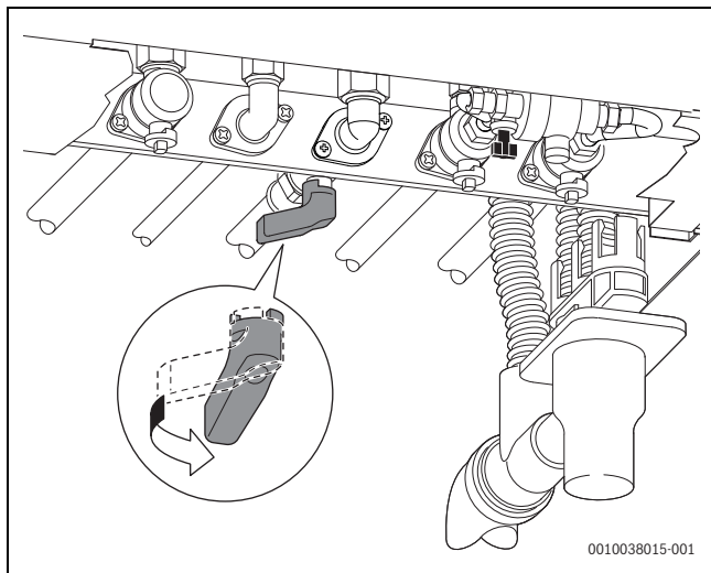
Fig. 6 Apertura del rubinetto del gas
