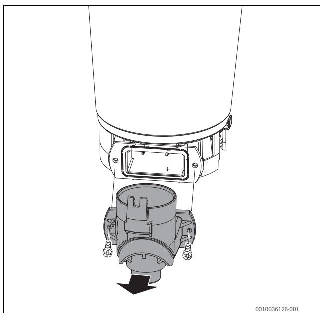
Fig. 61 Apertura dell'apertura di ispezione
