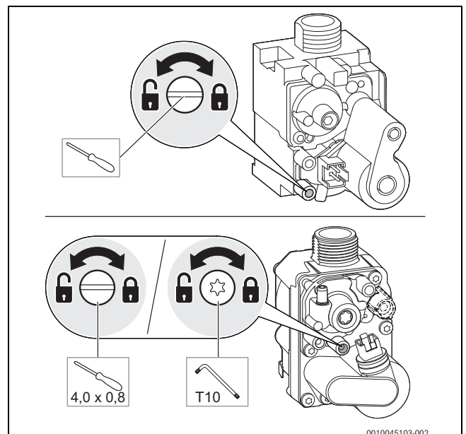
Fig. 45 Misurazione della pressione di collegamento del gas
