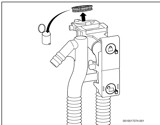
Fig. 65 Rimozione della guarnizione posta sul lato superiore del sifone per la condensa
