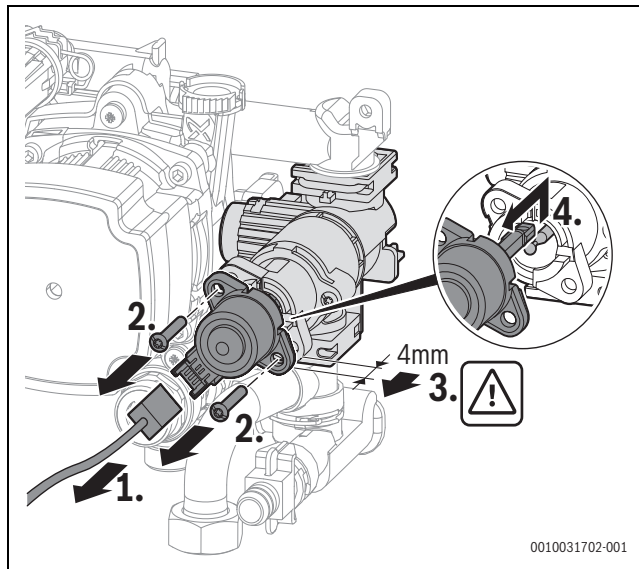
Fig. 81 Smontare il motore sulla valvola a 3 vie (variante con viti)
