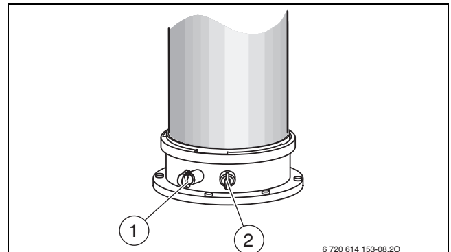
Fig. 49 Tronchetto di misurazione gas combustibili e tronchetto di misurazione per aria comburente
