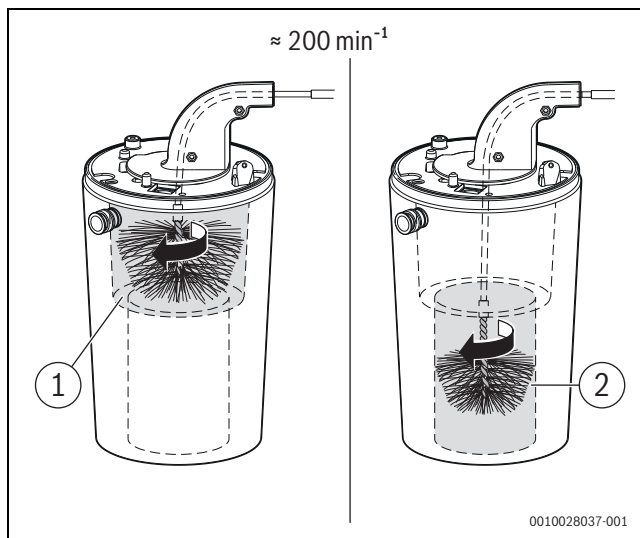
Fig. 60 Pulizia dello scambiatore primario (circa 200 \text{ min}^{-1} , solo rotazione destrorsa)
