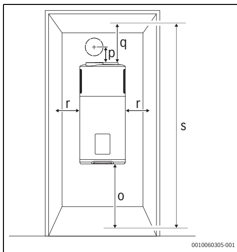
Fig. 9 Distanze minime senza struttura di supporto
