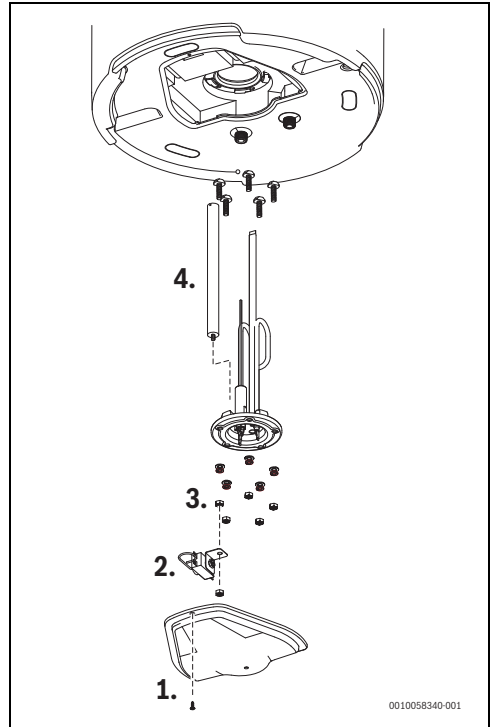
Fig. 31 Desmontaje del ánodo de magnesio
