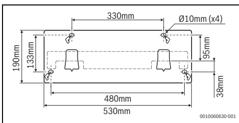
Fig. 11 Régua de fixação
