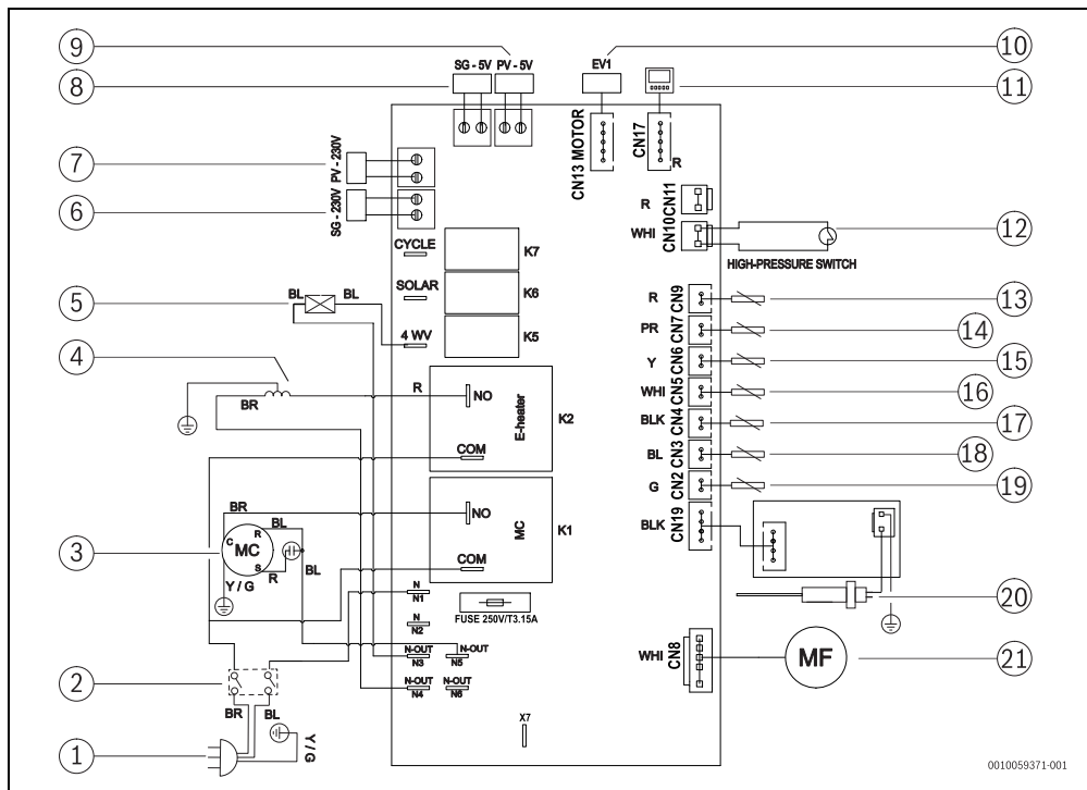
Fig. 33 Diagrama elétrico
