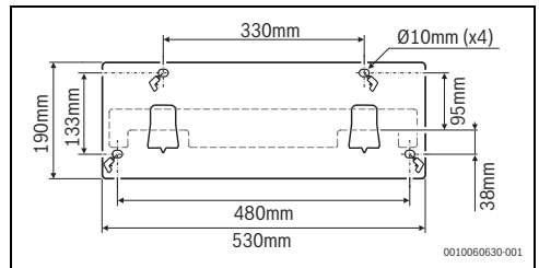
Fig. 11 Listón de fijación
