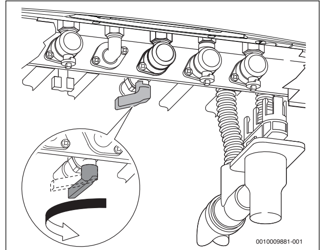
Fig. 2 Apertura del rubinetto del gas
