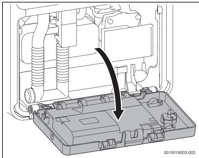
Fig. 28 Ribaltare verso il basso la scheda elettronica
