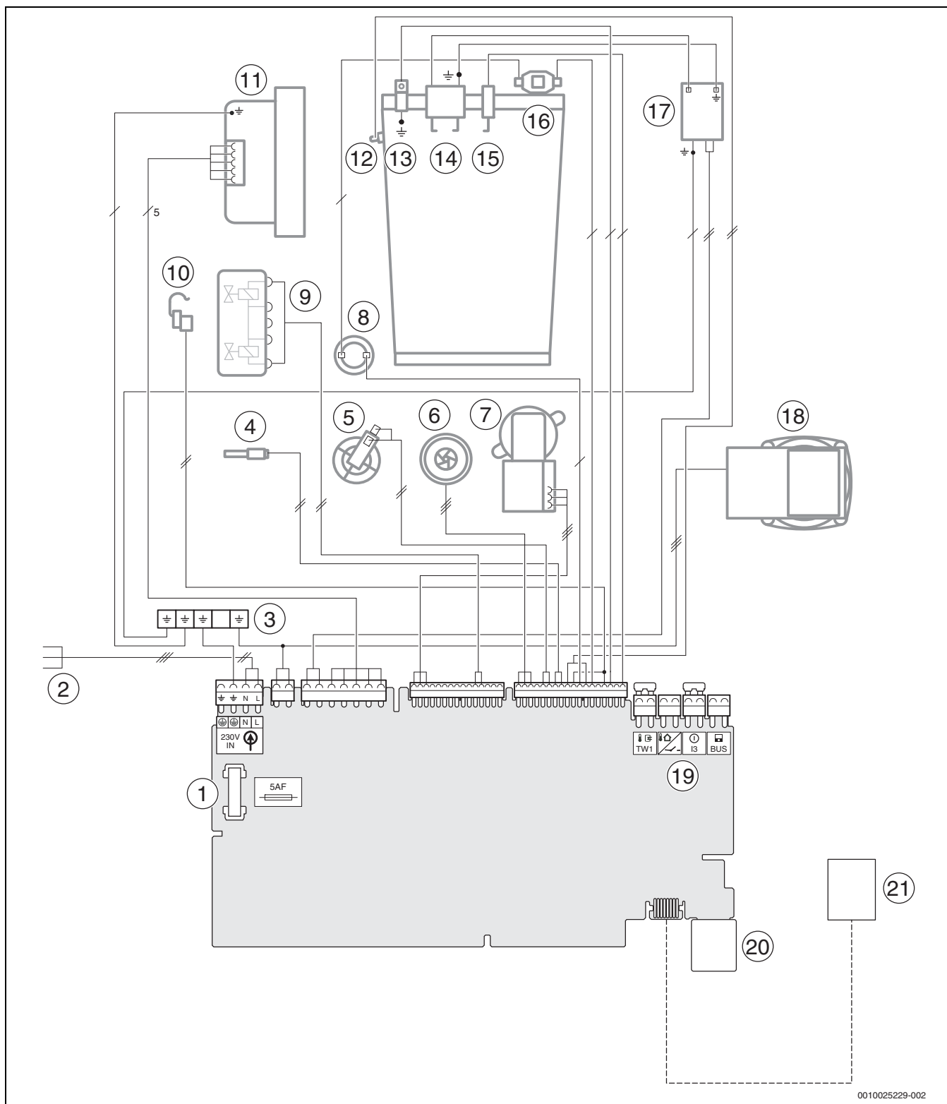
Fig. 73 Cablaggio elettrico
