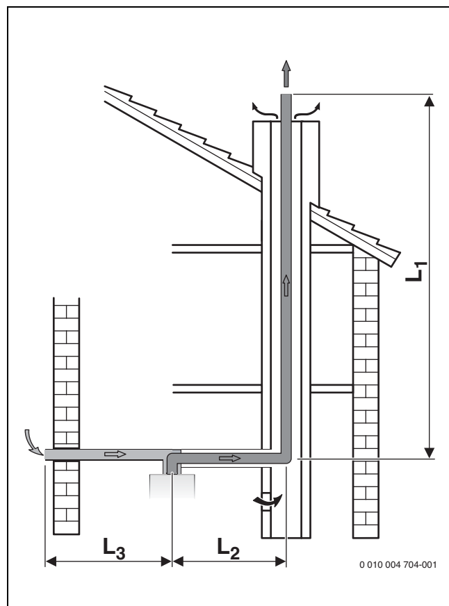
Fig. 10 Condotta di scarico combusti tramite cavedio secondo C 53
