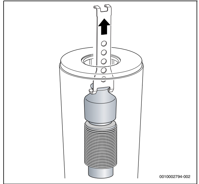
Fig. 47 Estrazione del deviatore di fiamma superiore
