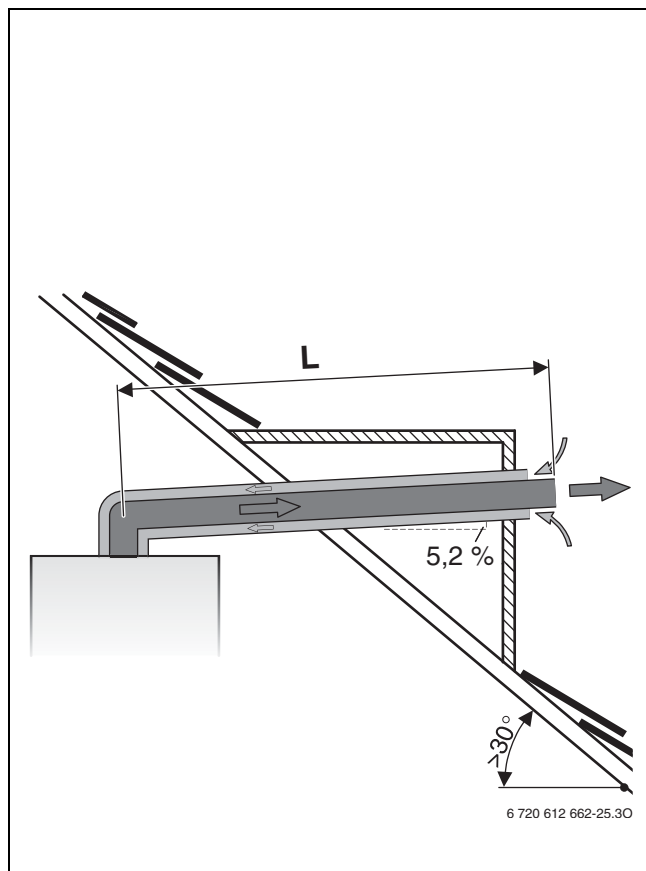
Fig. 12 Passaggio gas combusti orizzontale secondo C 13
