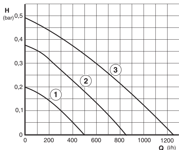
Fig. 22 Curve caratteristiche delle pompe
