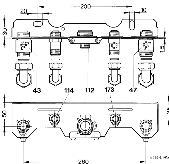
Fig. 5 Piastra di allacciamento e montaggio
