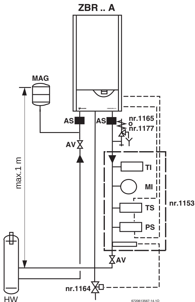
Fig. 13 Schema funzionale
