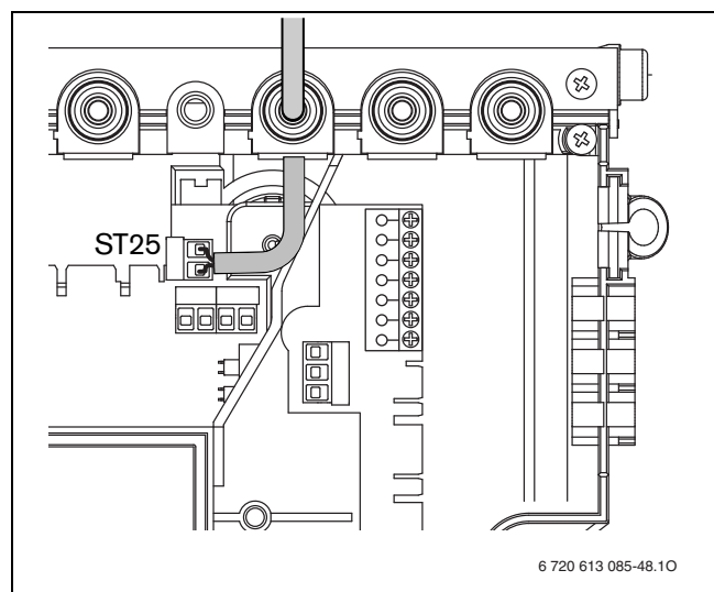
Fig. 29 Collegamento pompa di ricircolo sanitario
