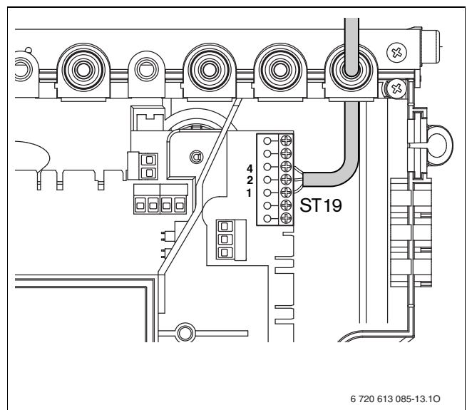
Fig. 26 Collegamento cronotermostati ambiente Junkers, a 24 V
