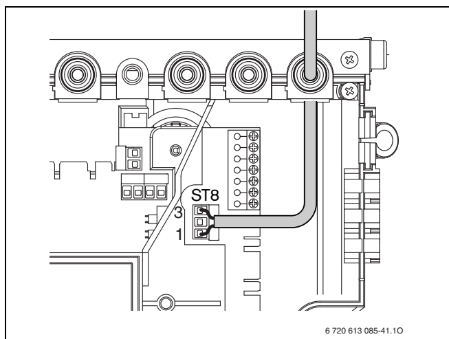
Fig. 28 Collegamento termostato del bollitore
