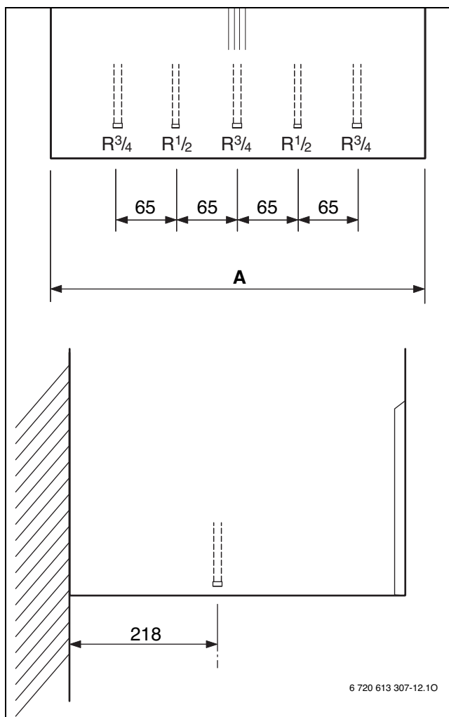
Fig. 17 Misure dei collegamenti
