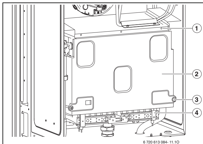
Fig. 58 Aprire il bruciatore
