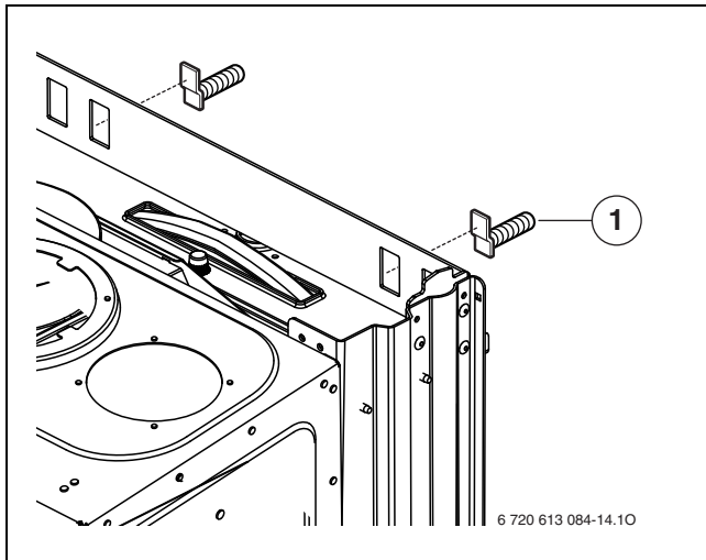
Fig. 13 Aggancio dell'apparecchio
