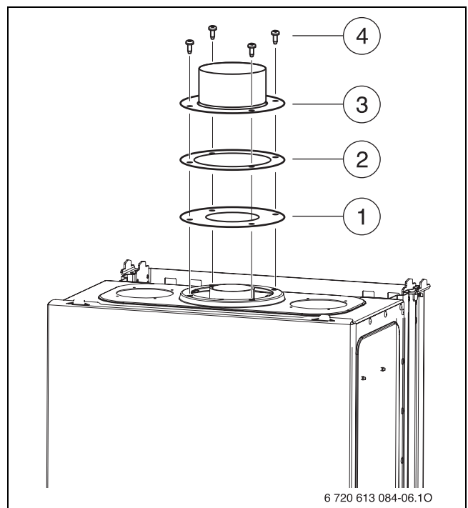
Fig. 16 Fissaggio dell'adattatore per aspirazione aria/scarico combusti
