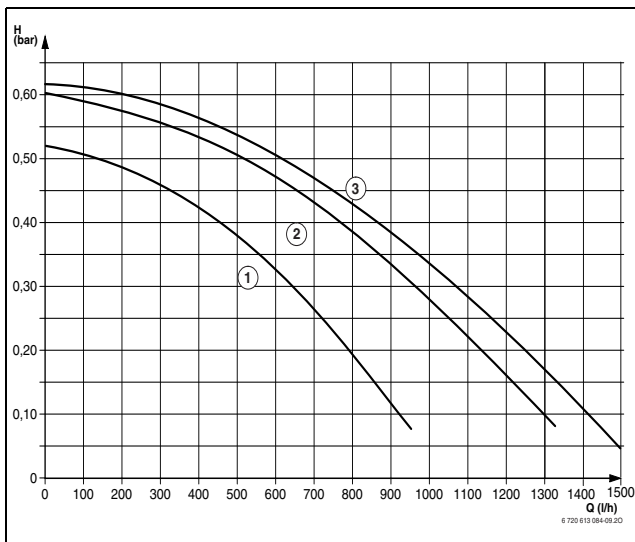
Fig. 43 Curves caratteristiche dei circolatori in ZWC 35-3 (senza piastra d'installazione)
