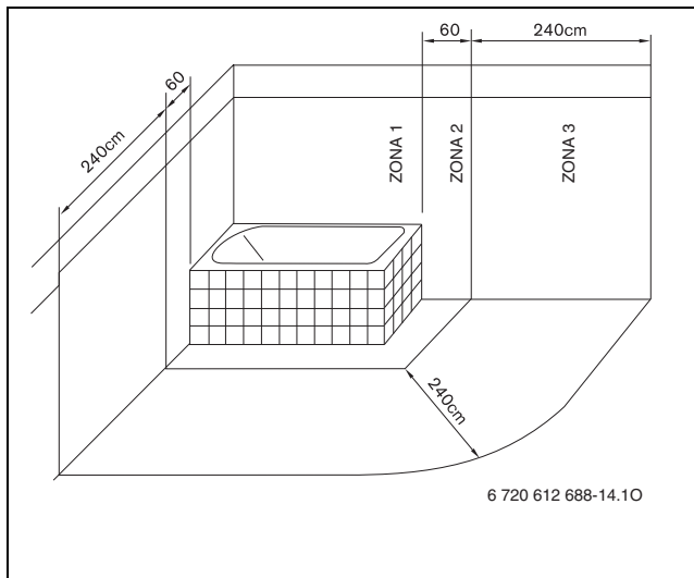
Fig. 18 Rappresentazione della Zona 3 (CEI 64-8)
