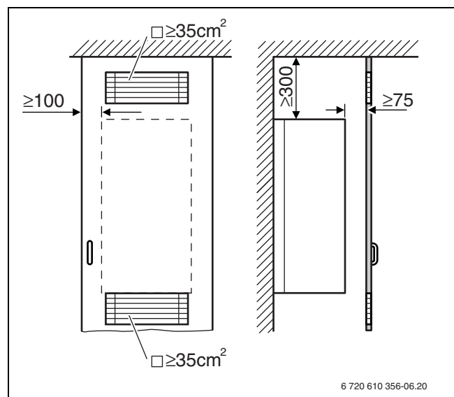
Fig. 6 Griglie di aerazione obbligatorie, in caso d'installazione in armadio copricaldaia
