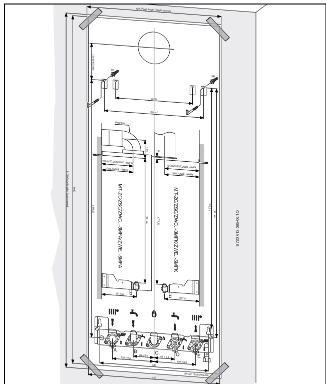
Fig. 7 Dima di preinstallazione
