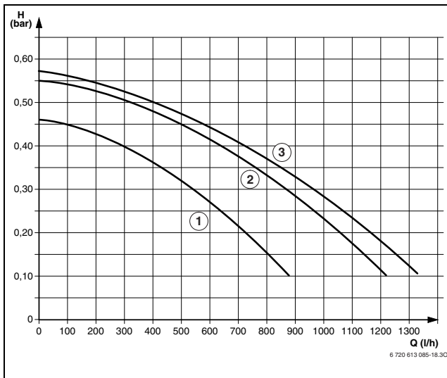
Fig. 42 Curves caratteristiche dei circolatori in ZWC/ZSC 28-3 (senza piastra d'installazione)
