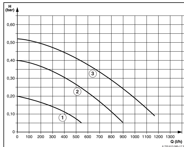
Fig. 41 Curva caratteristica dei circolatori in ZWC/ZSC 24-3 (senza piastra d'installazione)
