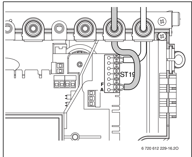
Fig. 25 Allacciamento della sonda esterna
