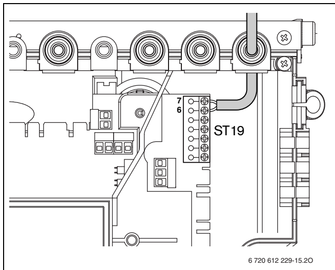
Fig. 24 Allacciamento del regolatore
